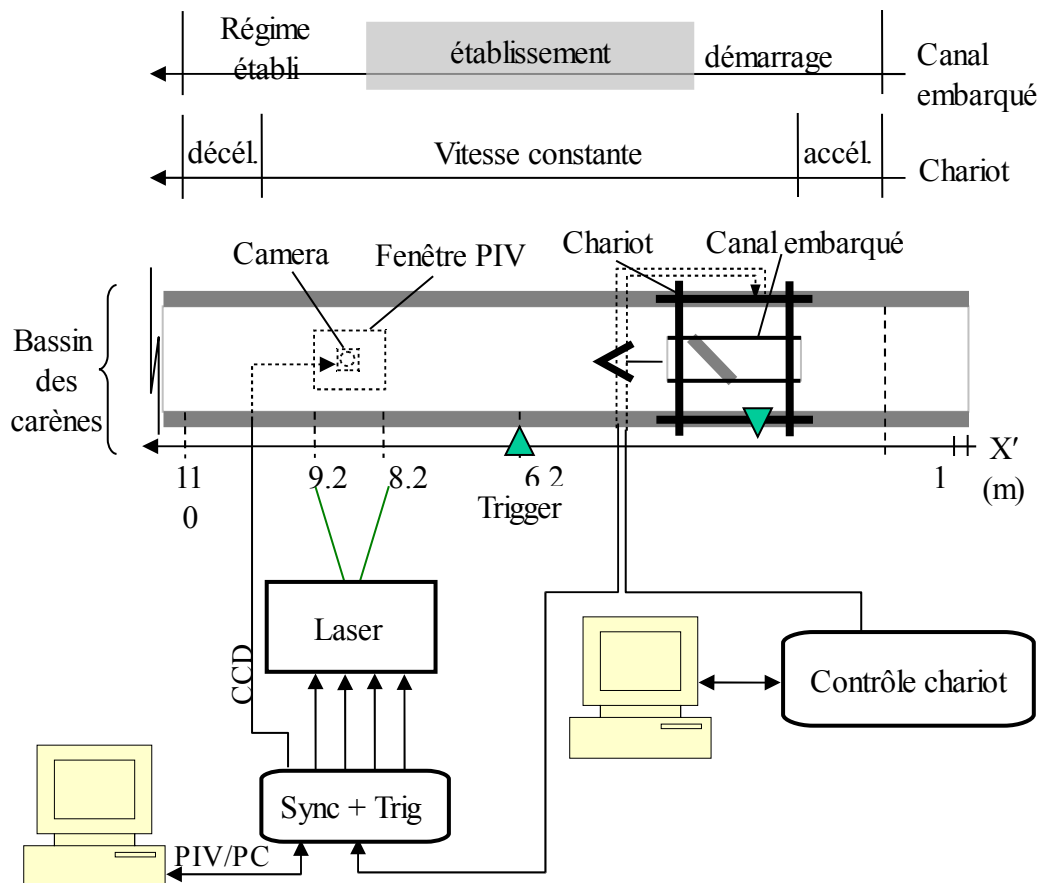
Figure 2: Dispositif PIV synchronisé avec le déplacement du chariot
