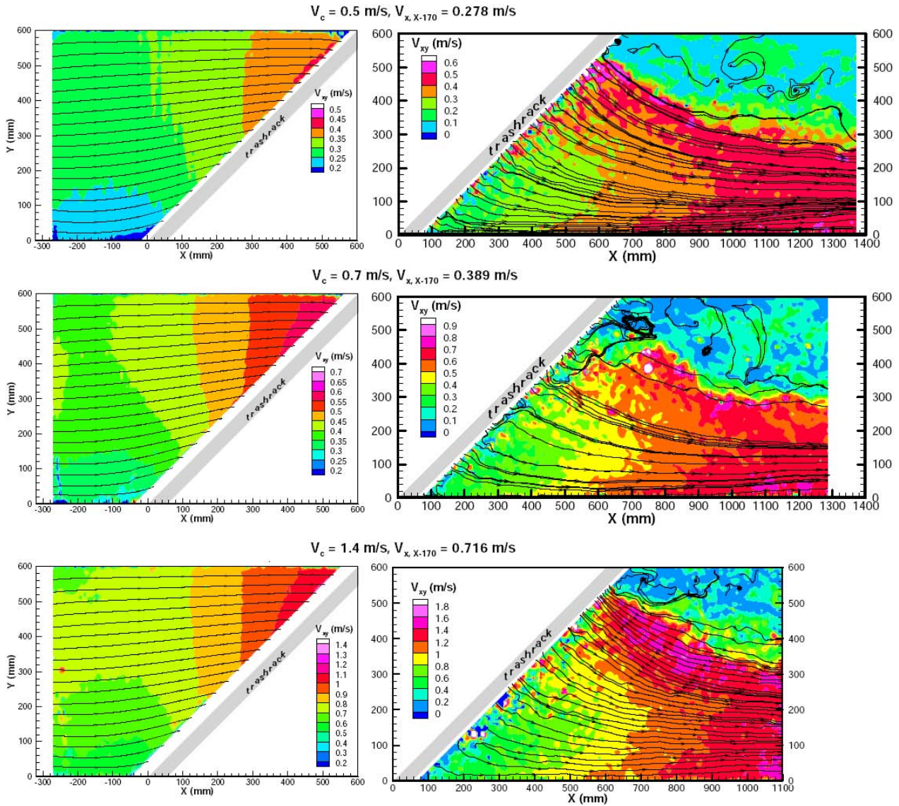
Figure 4: Champs de vitesses instantanées reconstruits en amont et en aval d'un plan de grille à profils standards orienté à 45° pour un écartement e=20\text{mm} . V_c=0.5;0.7;1.4\text{m/s} .
