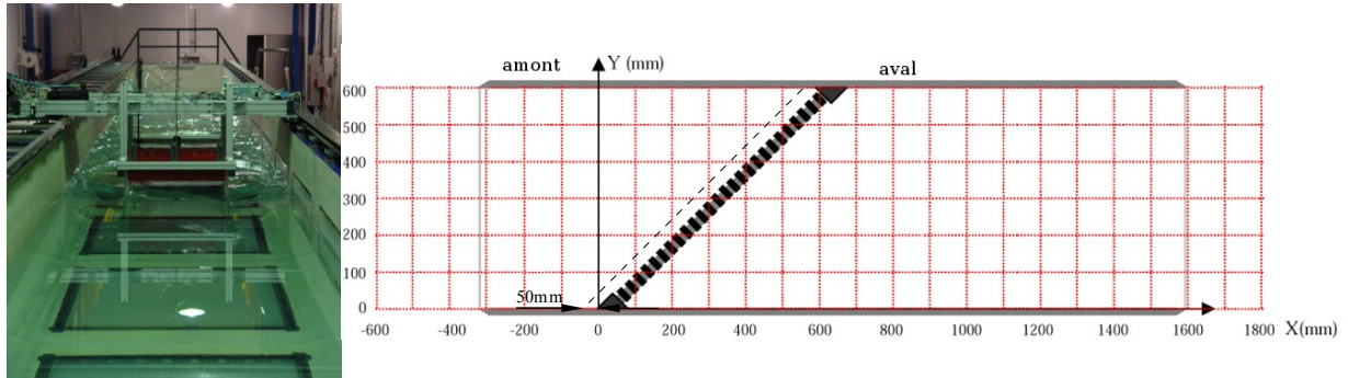
Figure 1: Aperçu et dimensions en plan du canal embarqué ; système de coordonnées associé et ligne de mesure des vitesses d'approche.
