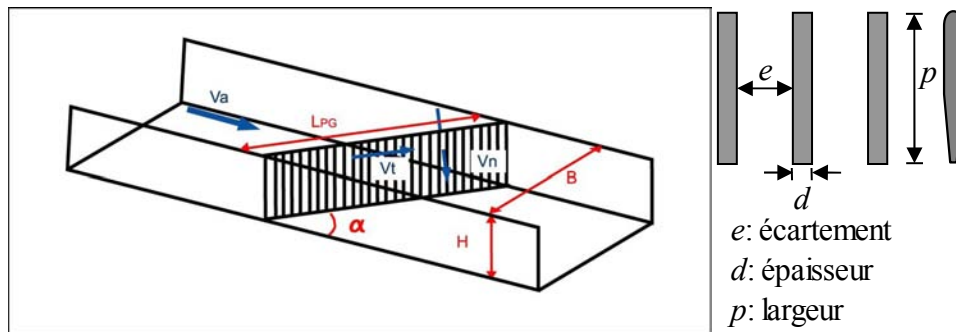
Figure 1 : Plan de grille orienté par rapport à un écoulement incident et configurations de grilles étudiées
