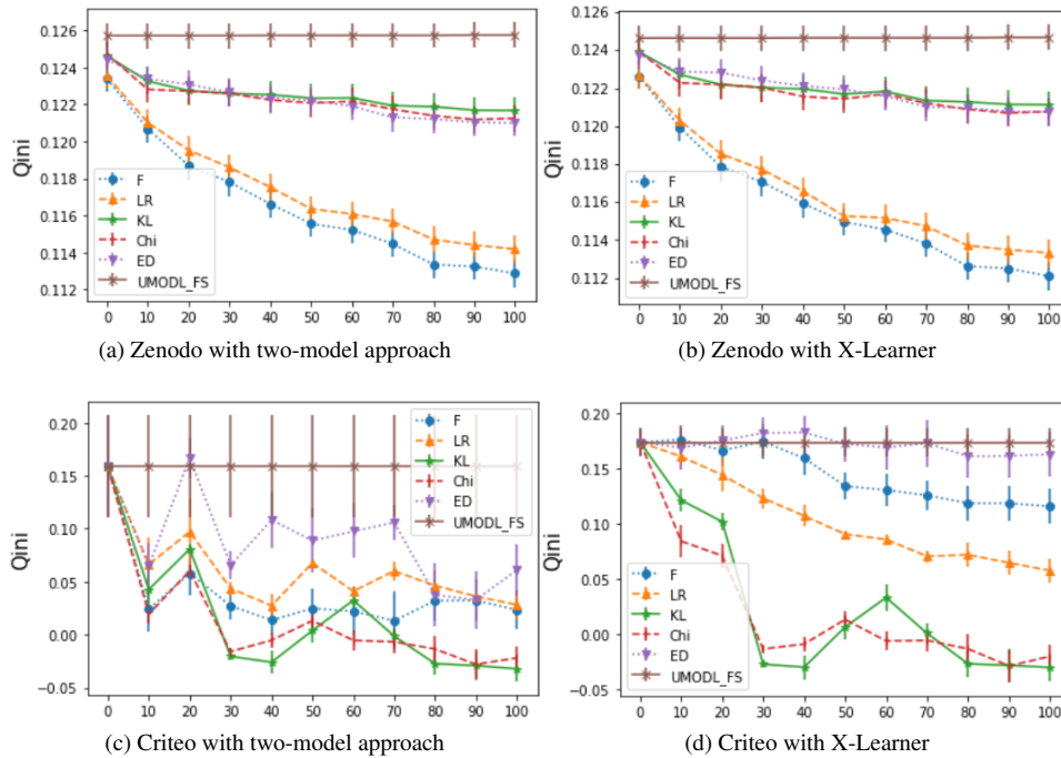
FIG. 2 – Moyenne de q_{ini} et sa variance en fonction du nombre de variables de bruit ajoutées. L'axe des X indique le nombre total de variables bruit ajoutées. L'axe Y représente les valeurs de q_{ini} obtenues par les modèles d'uplift.
