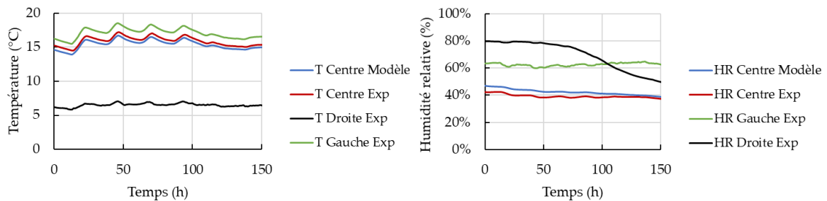
FIGURE 1. Pierre de Tuffeau et laine de bois du côté froid (type ITE).
