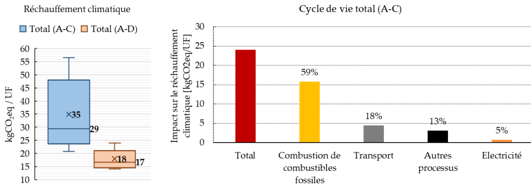
FIGURE 2. À gauche : ACV des 8 maçonneries ; à droite : principaux flux contributeurs (ex. : Tuffeau)
