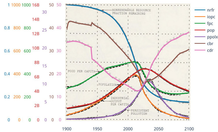
FIG. 1 – Reproduction de la Figure 7.7 de Meadows et al. [3]. Les courbes colorées ont été générées par notre framework et superposées au tracé original du livre.
