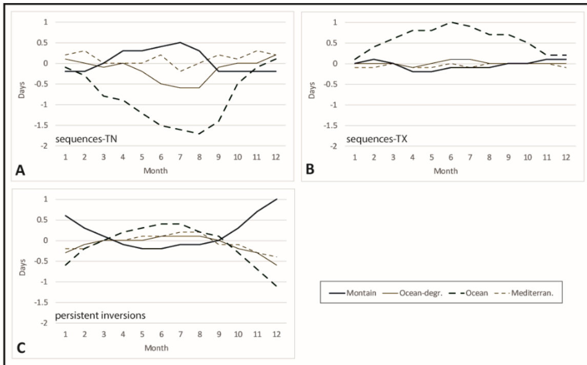
Figure 7. Deviations from the monthly average of inversion sequences and duration for each of the four climates (mountain, pure oceanic, degraded oceanic, and Mediterranean) and the twelve months of the year. Écarts par rapport à la moyenne des séquences et de la durée des inversions pour chacun des quatre climats (montagnard, pur océanique, océanique dégradé et Méditerranéen) et des 12 mois de l'année.
