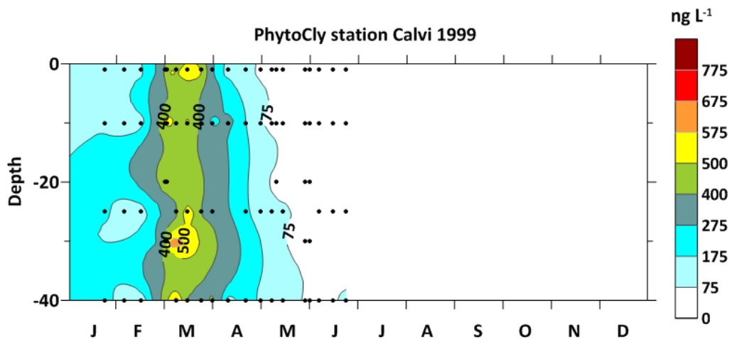
Figure 30. Évolution saisonnière de la Tchl a (mesures HPLC; en \text{ng}\cdot\text{L}^{-1} ) à la station PHYTOCLY entre janvier et juin 1999. Mesures de surface (A ; 5-6 prélèvements par semaine) et distribution verticale de la surface au fond (B ; 40 m, profils hebdomadaires, 4-5 profondeurs ; adapté de Goffart et al. 2015).
