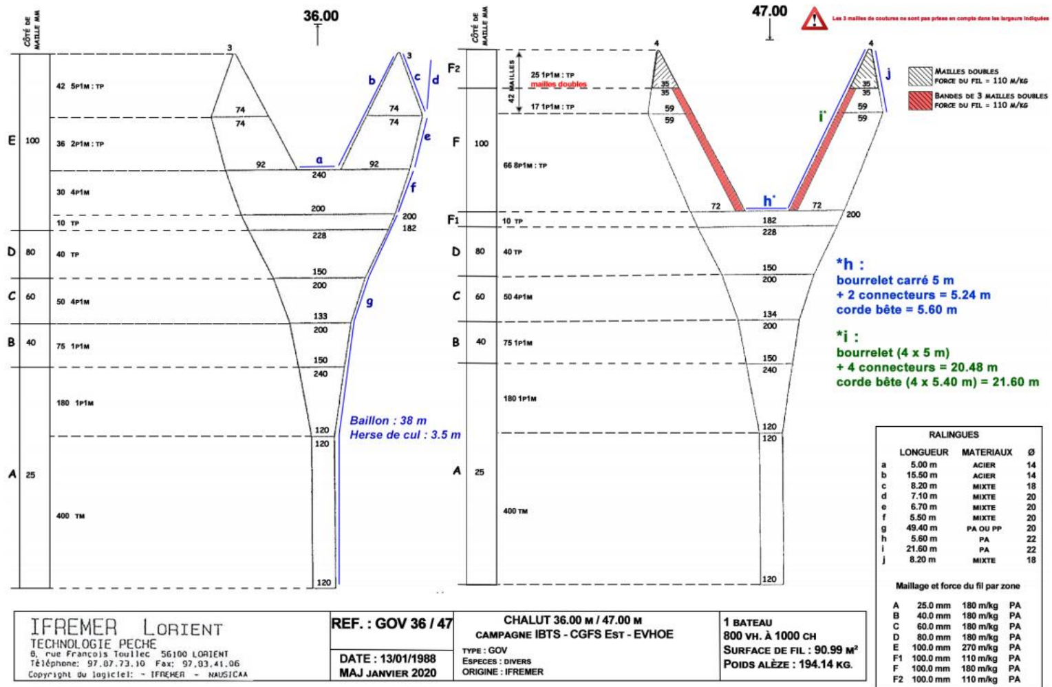
Figure 4 : Plan des faces du dessus et du dessous du châli GOV 36/47 utilisé lors des campagnes CGFS, EVHOE et IBTS. Le Roy (2018). Manuel Technique GOV 36/49 Mission CGFS Partie Ouest
