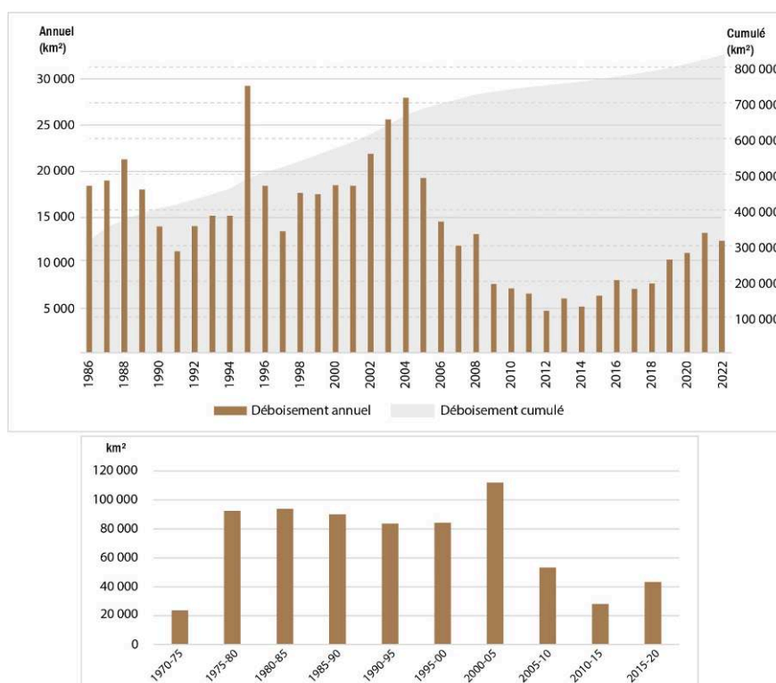
Illustration 6 - Le rythme de la déforestation en Amazonie brésilienne, 1986-2021
