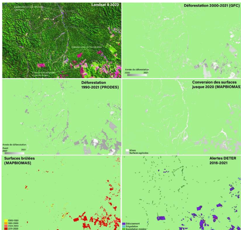
Illustration 8 - Comparaison des aires déboisées détectées par le PRODES, MAPBIOMAS, la GFC et le DETER sur une zone d'Amazonie brésilienne
