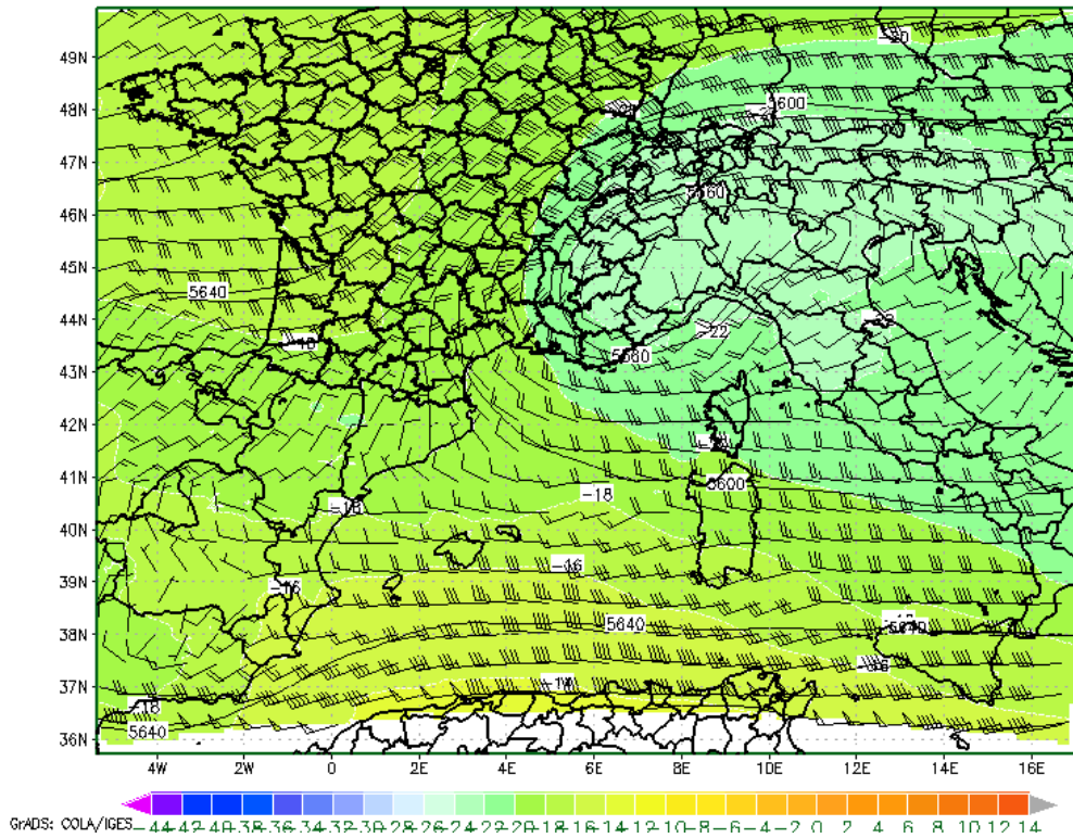
Figure 75 : Vents (nds) et température (deg.C plage de couleur) à 500hPa le 24 octobre 2007 à 18h
