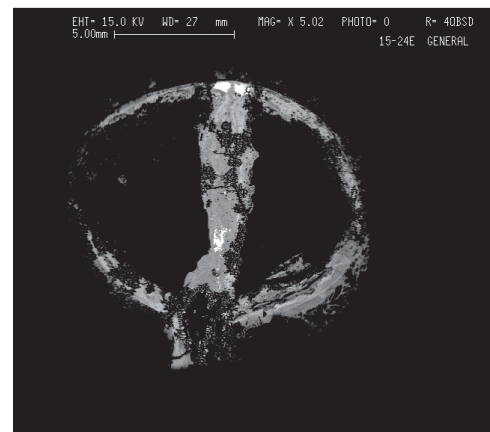
Fig. 6. Imagen metalográfica del apéndice de una fíbula serpentiforme de hierro (sección) obtenida por microscopía electrónica de rastreo (SEM) en modalidad BSE. Se trata de una esfera hueca insertada en un eje. En el extremo superior (zona blanca) se detectan restos de una sutura de cobre.
