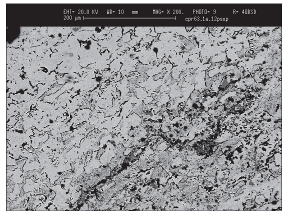
Fig. 5. Imagen metalográfica de la hoja de un cuchillo de hierro obtenida por microscopía electrónica de rastreo (SEM) en modalidad BSE. Se observa que el grado de acericación varía.
