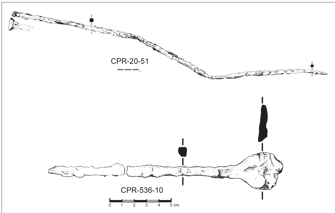
Fig. 4. Asadores férricos de Can Piteu – Can Roqueta, Sabadell.
