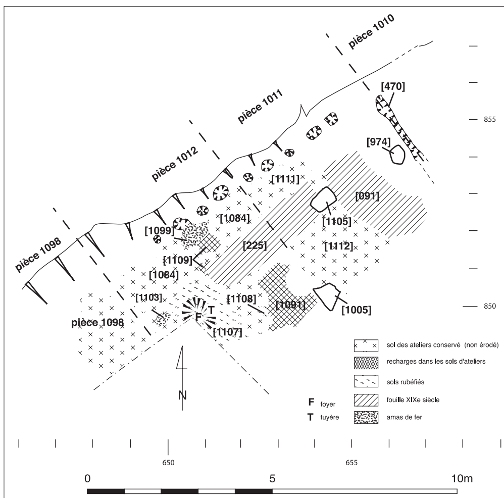
Fig. 2. Plan schématique de l'ensemble des structures conservées. DAO D. Beuscher.
