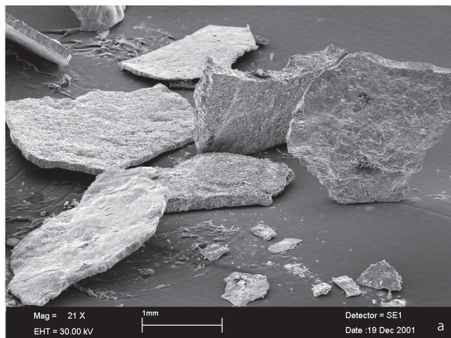
Fig. 5a. Battitures de type plaquettes ; b. Battitures de type sphéroïdes (photos D. Dungworth).
