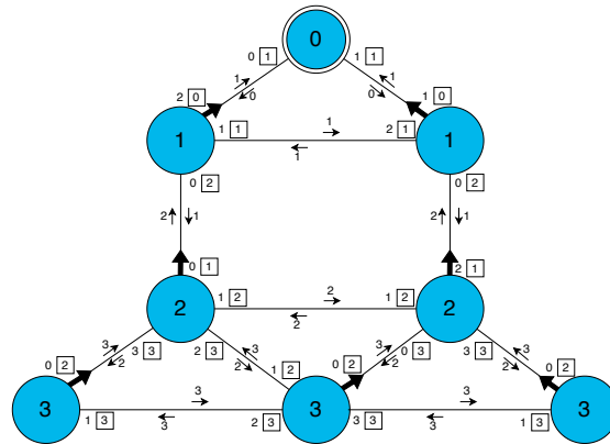
FIGURE 5 – Exemple d'état légitime de l'algorithme autostabilisant de calcul d'arbre couvrant. Les flèches épaisses représentent les pointeurs parent. Pour chaque processus p_i , chaque couple « j \boxed{k} » représente son numéro de port j et la valeur de distance k associée. Les flèches fines et leurs valeurs associées représentent des messages en transit.
