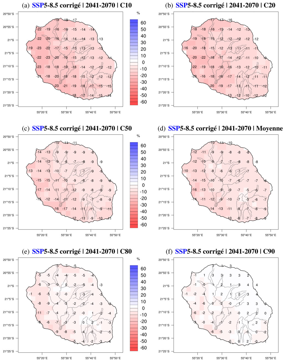
FIGURE 6.71 – Similaire à la figure 6.69 mais pour le scénario SSP5-8.5 en milieu de siècle.
