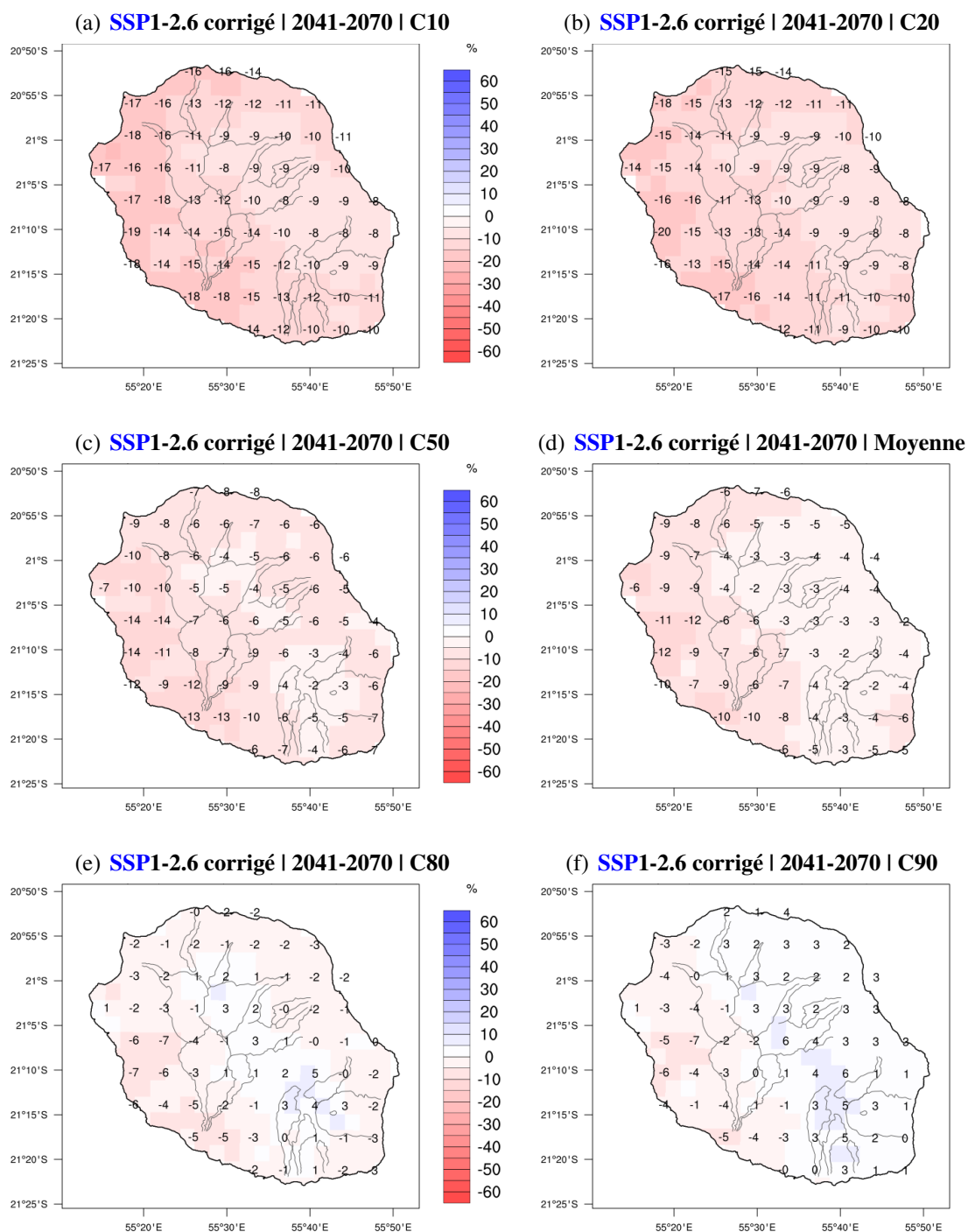
FIGURE 6.69 – Centiles des anomalies (en % par rapport à la normale 1981-2010) des cumuls annuels moyens de précipitations sur La Réunion pour un ensemble de 22 modèles globaux CMIP6 pour le scénario SSP1-2.6 en milieu de siècle, après descente d'échelle statistique.
