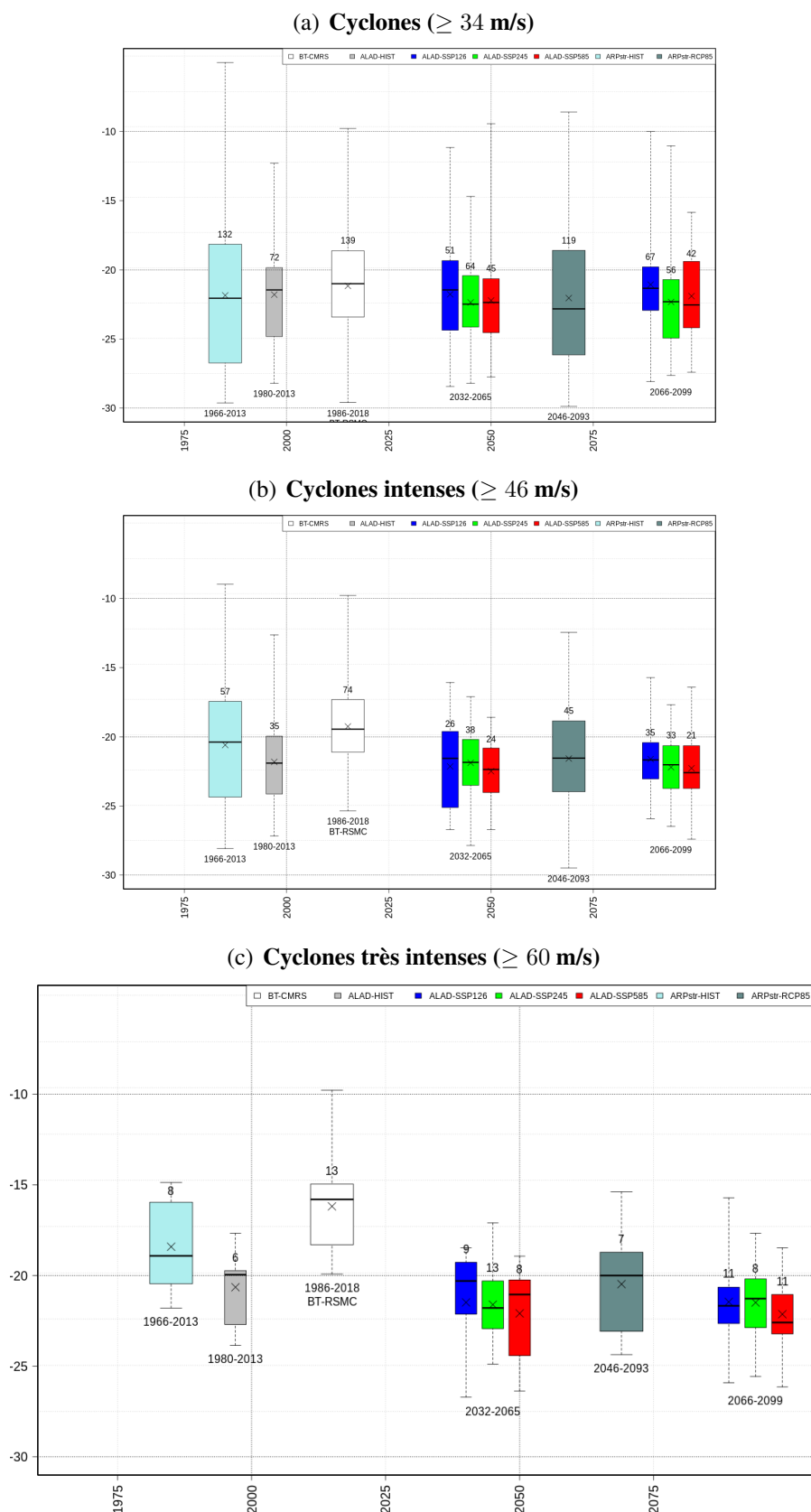
FIGURE 6.20 – Evolution de la latitude du maximum d'intensité cyclonique sur la période 1965-2100 par catégorie d'intensité ((a) à (c)) dans les simulations ALADIN (3 scénarios SSP) et ARPEGE-str (scénario RCP8.5). Les valeurs de la Best track sont affichées pour référence. Les modèles ont été préalablement corrigés de leurs biais en intensité. Les boîtes à moustaches mettent en valeur la médiane C50 (trait), la moyenne (croix), les 1 er et 3 ème quartiles i.e. les centiles C25 et C75 (contours des boîtes), et les valeurs minimales et maximales.
