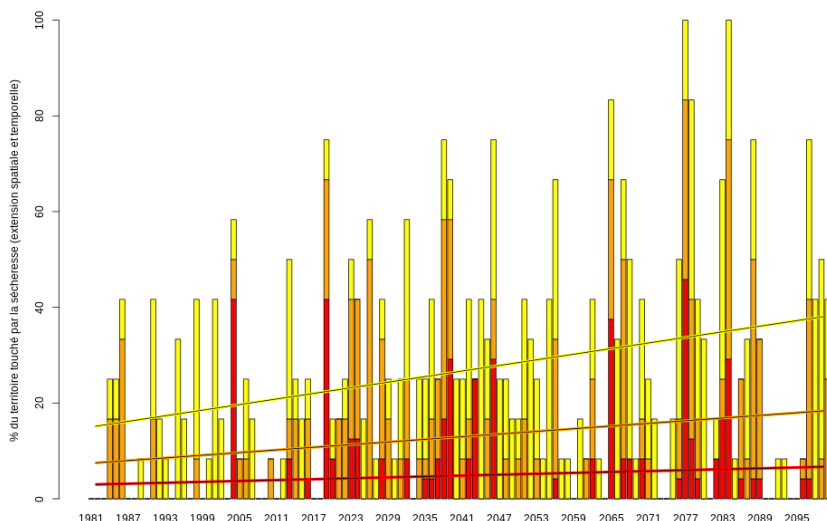
FIGURE 6.56 – Evolution temporelle sur la période 1981-2100 de l'indice sécheresse sur Mayotte selon le modèle régional ALADIN pour le scénario SSP5-8.5 , après correction des biais : pourcentage du territoire touché par la sécheresse. Légende similaire à la figure 6.51.
