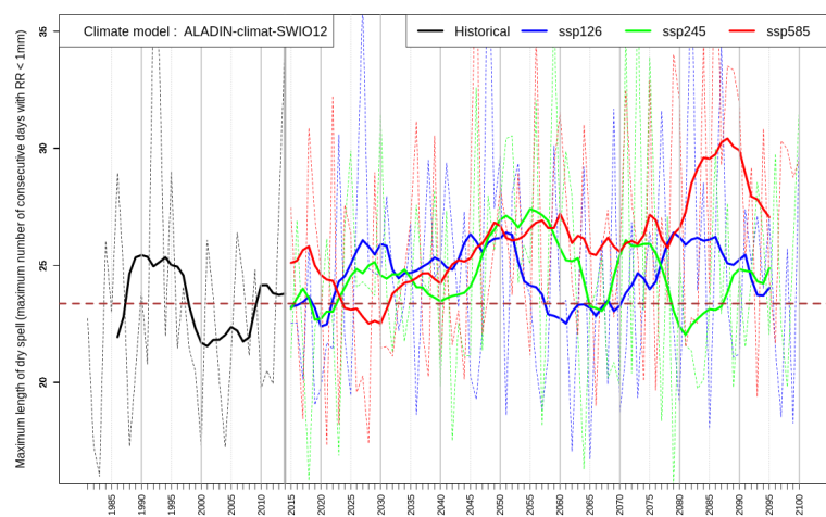
FIGURE 6.50 – Evolution temporelle du nombre annuel maximal de jours secs consécutifs (indicateur CDD défini au tableau 6.1) prévu par ALADIN sur l'île de La Réunion jusqu'en 2100 pour 3 scénarios SSP, après correction des biais. La ligne horizontale tiretée situe la moyenne de référence 1981-2010. Un lissage sur 10 années glissantes est réalisé pour atténuer la variabilité interannuelle.
