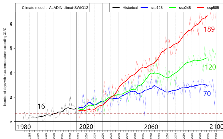
FIGURE 6.49 – Evolution temporelle du nombre de jours annuel où la température maximale simulée par ALADIN dépasse le seuil de 31°C sur Gillot, La Réunion, depuis la période passée 1981-2014 (en noir) jusqu'à l'horizon 2100 pour 3 scénarios SSP (couleurs), après correction des biais. La ligne horizontale tiretée situe la moyenne de référence 1981-2010. Les chiffres superposés au graphique indiquent les valeurs moyennes sur la période historique en noir et sur l'horizon de fin de siècle 2071-2100 en couleur dans chaque scénario. Un lissage sur 10 années glissantes est réalisé pour atténuer la variabilité interannuelle.
