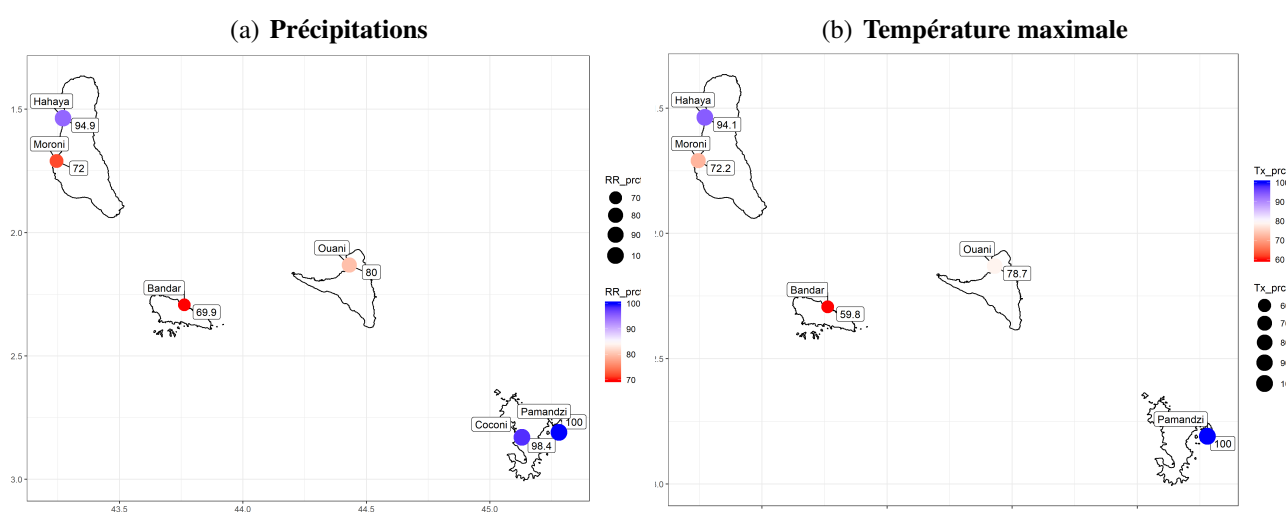
FIGURE 4.27 – Sélection des stations de mesures climatologiquement exploitables sur l'archipel des Comores en fonction du taux de données disponibles (en %) pour la période 1981-2010 pour les variables (a) précipitations (RR) et (b) température maximale (Tx).
