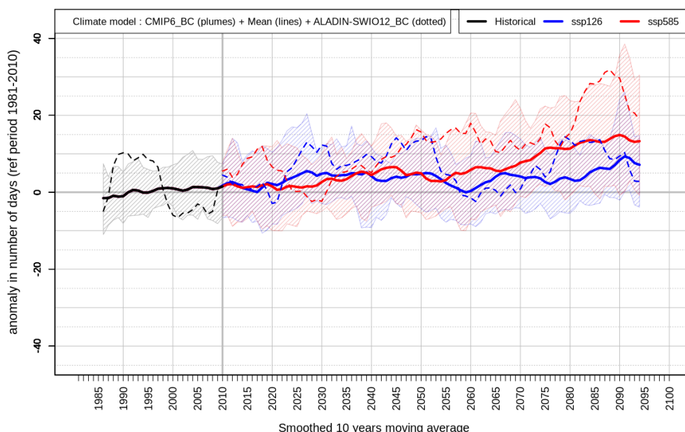
FIGURE 6.73 – Evolution temporelle sur la période 1981-2100 du nombre maximal de jours secs consécutifs par an (indicateur CDD défini au tableau 6.1) sur La Réunion selon 22 modèles globaux de CMIP6 corrigés par descente d'échelle statistique pour 2 scénarios SSP (enveloppes de couleur et moyenne multi-modèle en traits continus) et selon le modèle régional ALADIN (traits pointillés) après correction des biais. L'historique est en noir et les projections pour 2 scénarios en couleurs. Les données représentées sont des moyennes glissantes sur 10 ans. Les enveloppes de couleurs délimitent les valeurs des centiles 10 à 90 (C10-C90) c'est-à-dire 80% de la distribution des 22 modèles CMIP6 et excluent les valeurs plus extrêmes (20% de la distribution).
