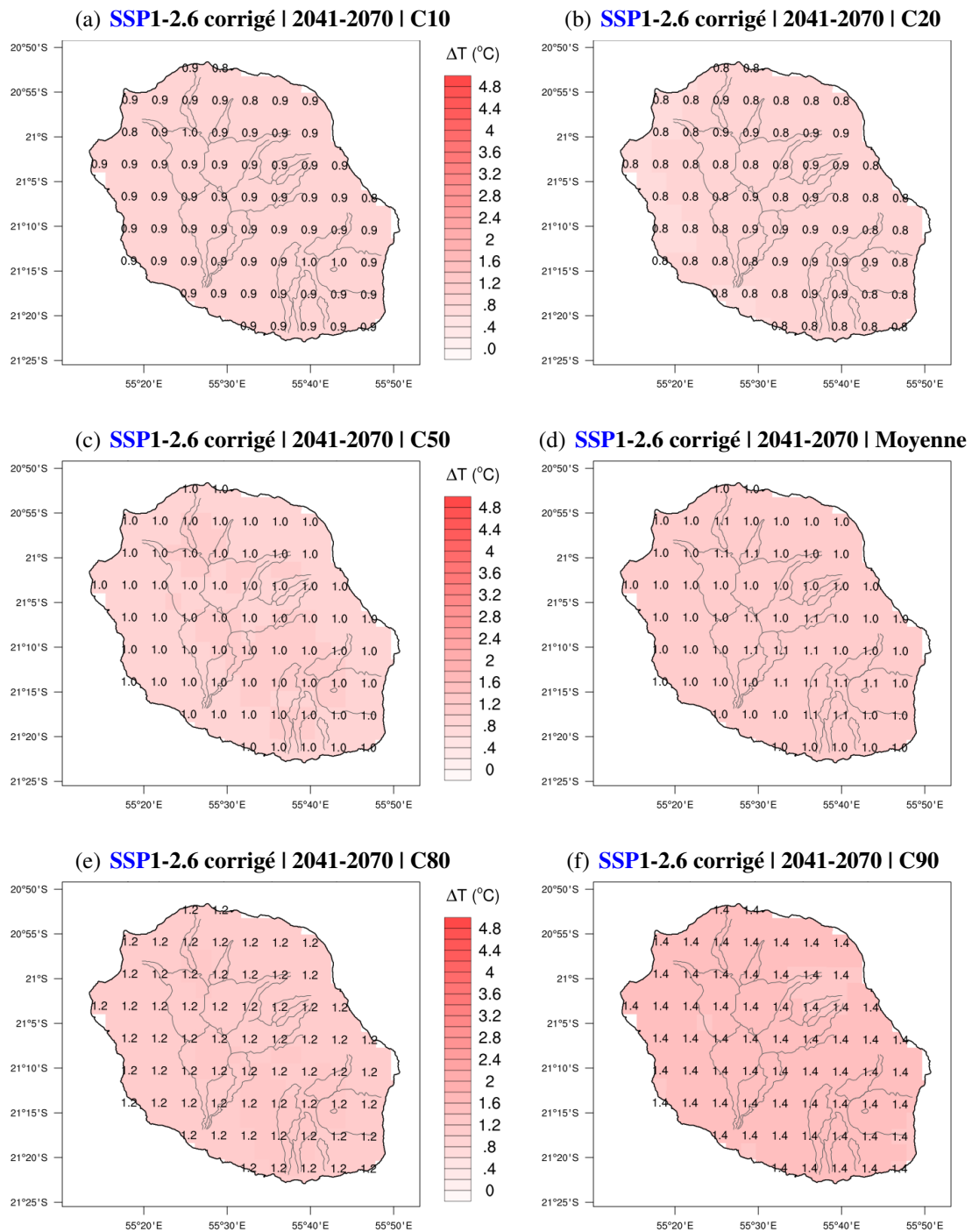
FIGURE 6.75 – Centiles des anomalies (en ^{\circ}\text{C} par rapport à la normale 1981-2010) de la température moyenne annuelle à +2 m sur La Réunion pour un ensemble de 22 modèles CMIP6 pour le scénario SSP1-2.6 en milieu de siècle, après descente d'échelle statistique.
