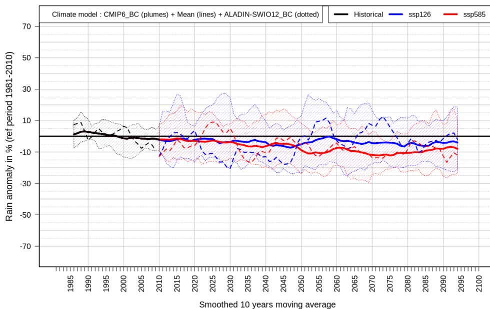
FIGURE 6.68 – Evolution temporelle sur la période 1981-2100 des anomalies du cumul annuel de précipitations (en % par rapport à la normale 1981-2010) sur La Réunion selon 22 modèles globaux de CMIP6 corrigés par descente d'échelle statistique pour 2 scénarios SSP (enveloppes de couleur) et selon le modèle régional ALADIN (traits pointillés) après correction des biais. L'historique est en noir et les projections pour 2 scénarios en couleurs. Les données représentées sont des moyennes glissantes sur 10 ans. Les enveloppes de couleurs délimitent les valeurs des centiles 10 à 90 (C10-C90) c'est-à-dire 80% de la distribution des 22 modèles CMIP6 et excluent les valeurs plus extrêmes (20% de la distribution).
