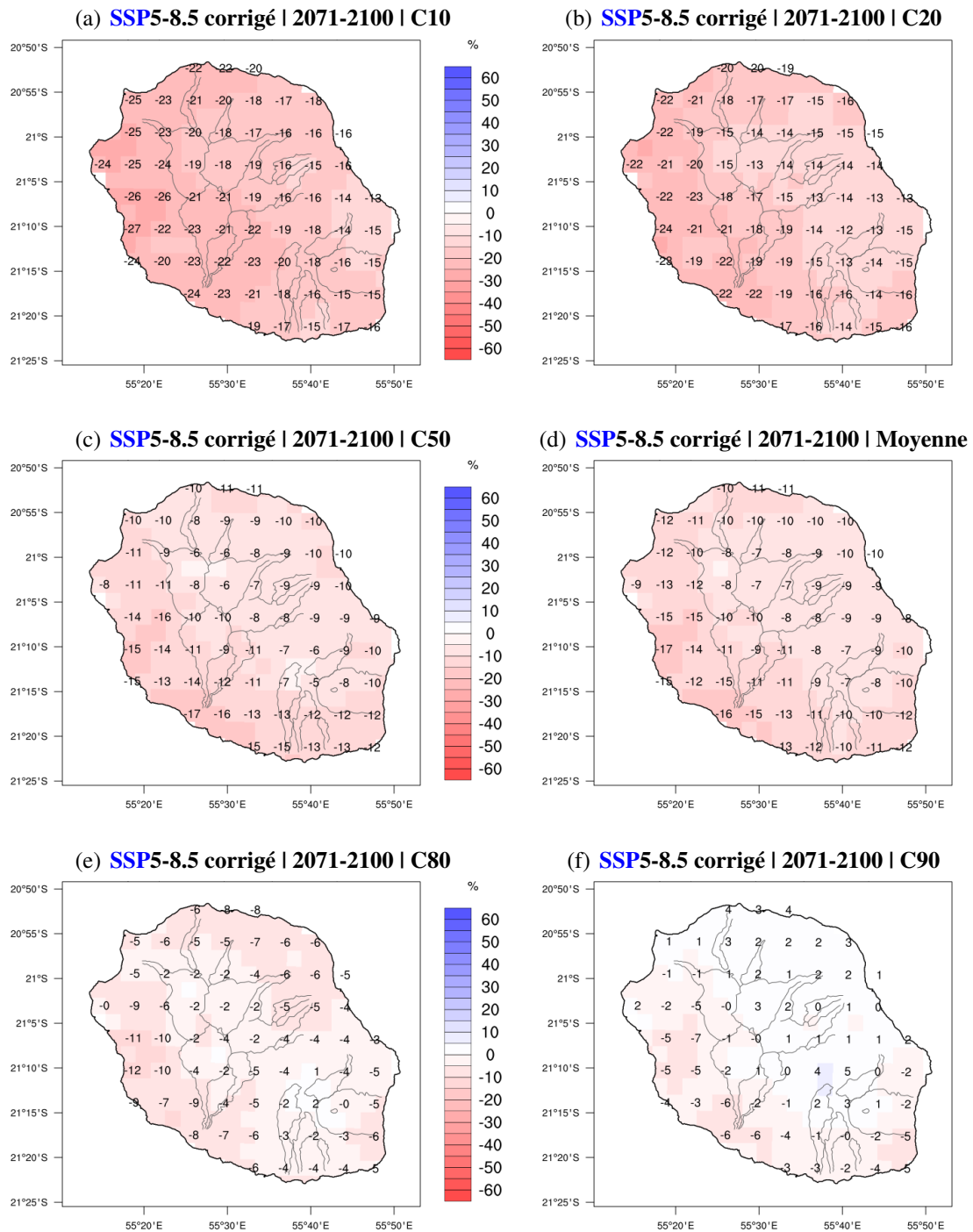
FIGURE 6.72 – Similaire à la figure 6.69 mais pour le scénario SSP5-8.5 en fin de siècle.
