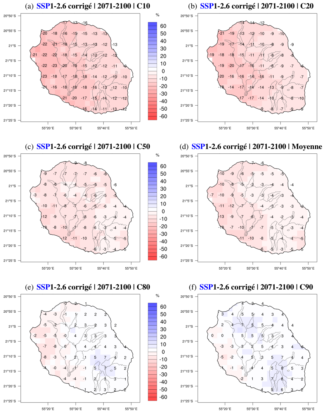
FIGURE 6.70 – Similaire à la figure 6.69 mais pour la fin de siècle.
