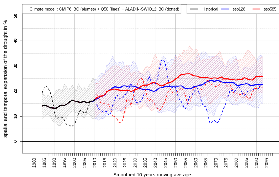
FIGURE 6.74 – Evolution temporelle sur la période 1981-2100 de l'indice sécheresse sur La Réunion selon 22 modèles globaux de CMIP6 corrigés par descente d'échelle statistique pour 2 scénarios SSP (enveloppes de couleur et moyenne multi-modèle en traits continus) et selon le modèle régional ALADIN (traits pointillés) après correction des biais : pourcentage du territoire touché par la sécheresse. Les valeurs peuvent évoluer chaque année entre 0 (aucune partie du territoire en sécheresse pluviométrique à aucun moment de l'année) et 100 (tout le territoire en sécheresse pluviométrique tout au long de l'année). L'historique est en noir et les projections pour 2 scénarios en couleurs. Les données représentées sont des moyennes glissantes sur 10 ans. Les enveloppes de couleurs délimitent les valeurs des centiles 10 à 90 (C10-C90) c'est-à-dire 80% de la distribution des 22 modèles CMIP6 et excluent les valeurs plus extrêmes (20% de la distribution).
