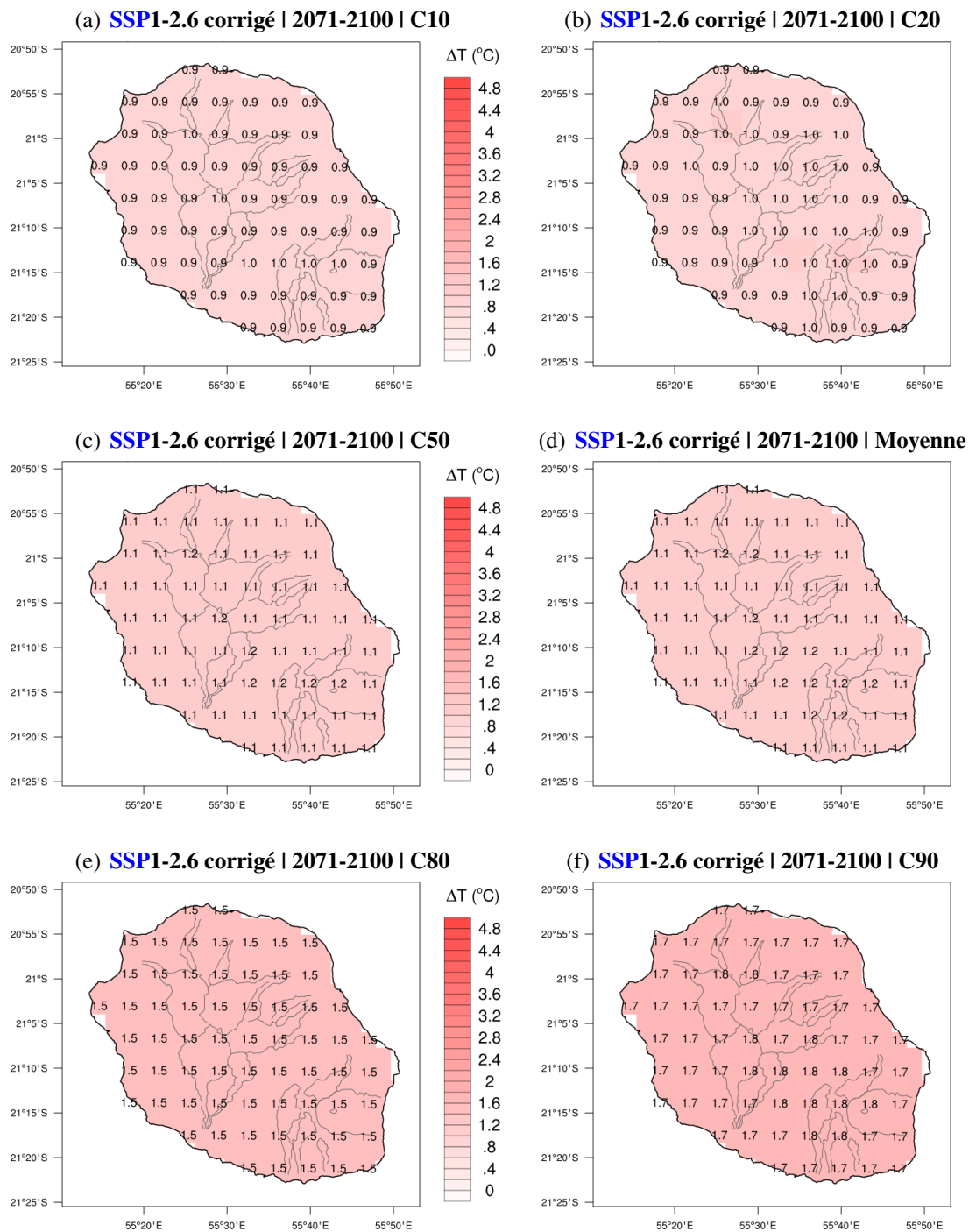
FIGURE 6.76 – Similaire à la figure 6.75 mais pour la fin de siècle.
