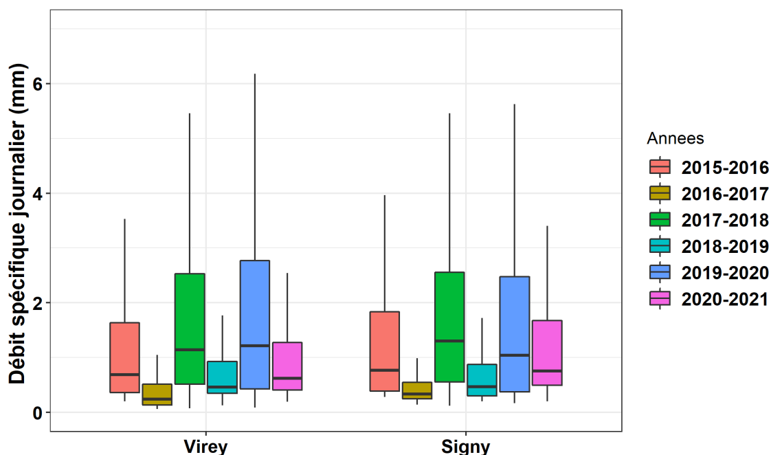
Figure 17 : Distribution en boxplot des débits spécifiques journaliers des stations amont (Virey) et aval (Signy) par année hydrologique.
