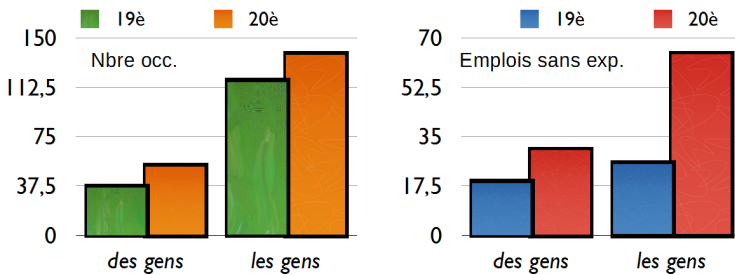
Graphique 4. Le nombre d'occurrences Graphique 5. Les emplois sans expansion
