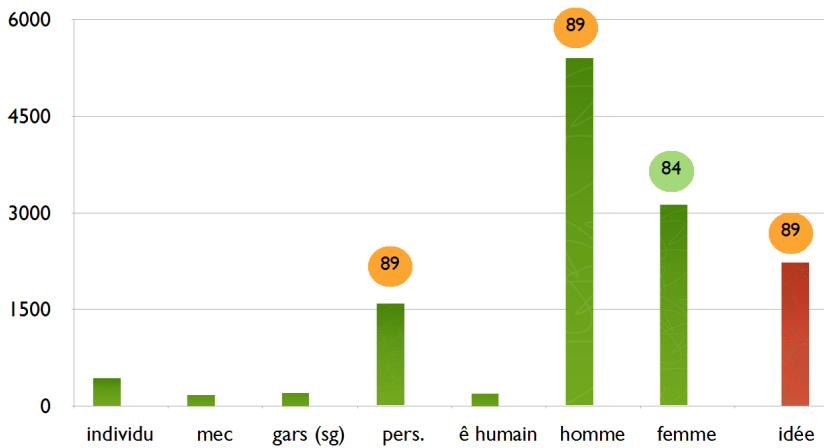
Graphique 1. Nombre d'occurrences et répartition dans les sous-corpus du CERF
