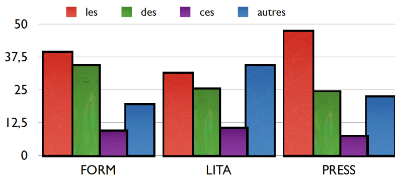
Graphique 3. Répartition des voisins de gauche de gens dans 3 sous-corpus du CERF
