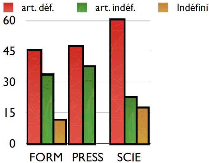
Graphique 2. Part des articles défini, indéfini et du déterminant indéfini avec individu
