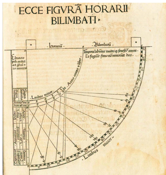
FIGURE 1 – Dessin donné par Stöffler en 1513 du cadran à double limbe.
