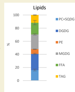
Chlorella vulgaris
