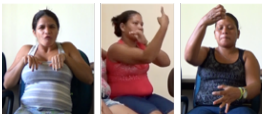
Figure 1 – Exemples de TP, TS et TTF, ici dans la LS du Marajó
