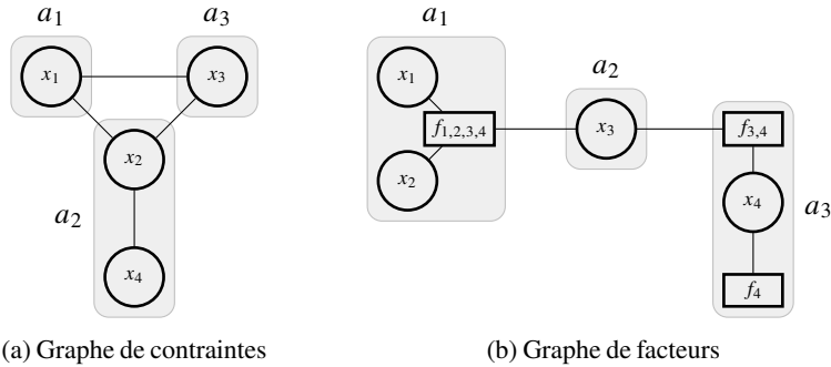
FIGURE 2.1 – Représentations graphiques pour les DCOPs
