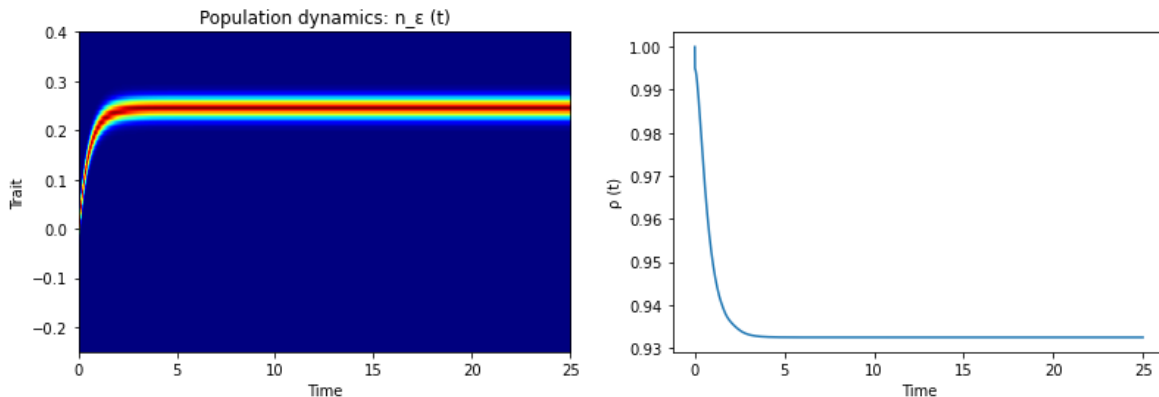
(A) Function n_\varepsilon(t, z)
