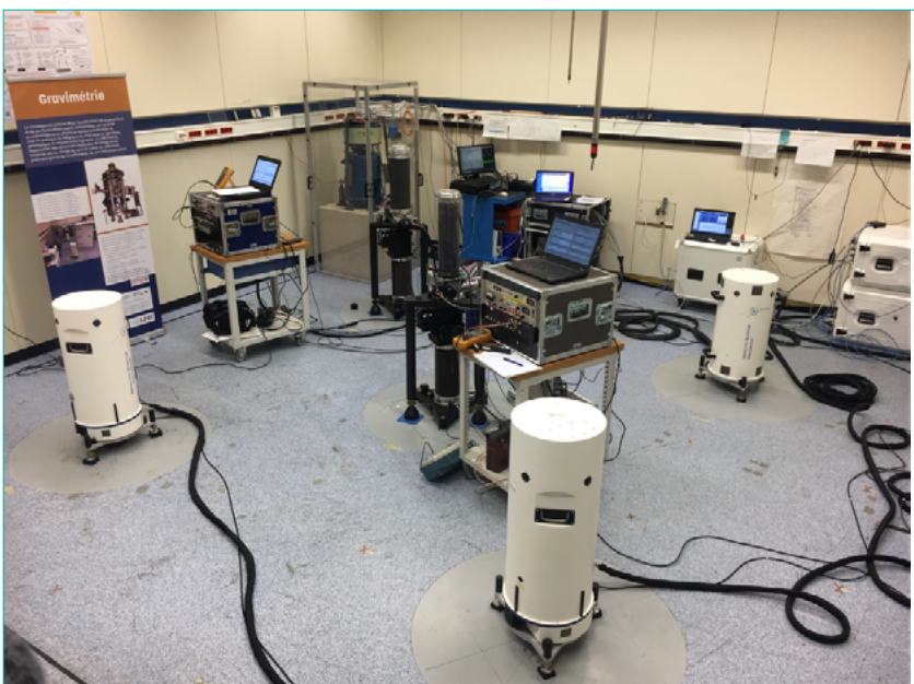
1 Comparaison des gravimètres absolus du Parc d'instruments national PGrav géré par l'Action spécifique gravimétrie. En blanc : AQG, en noir : FG5, au fond en bleu : iGrav. © Sébastien Merlet. Pour en savoir plus : https://www.resif.fr/blog/2022/10/24/comparaison-des-gravimetres-absolus-du-pin-pgrav/
