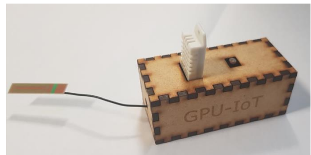
fig 3 : Objet connecté permettant de mesurer la qualité de l'environnement de travail
