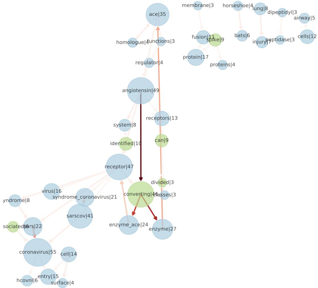
Figura 2 Grafo de conocimientos que representa las oraciones que contienen los vocablos coronavirus y angiotensin .
