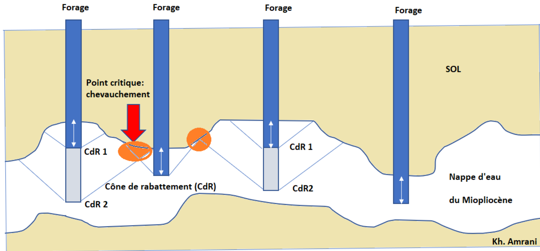
Figure 28 : schéma simplifié représentant le chevauchement du cône de dépression des forages approfondis de façon « non-concertée ». Ces comportements provoquent un rabattement spectaculaire de la nappe et pénalise tous les agriculteurs à proximité.
