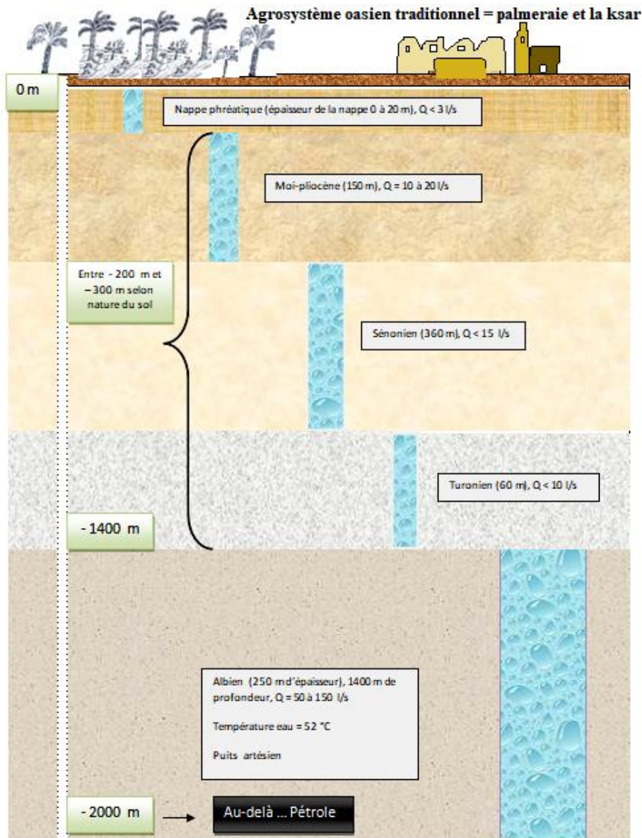
Figure 12 : Les différents aquifères sous les palmeraies de la cuvette de Ouargla (d'après données ANRH : Agence Nationale des Ressources Hydriques)
