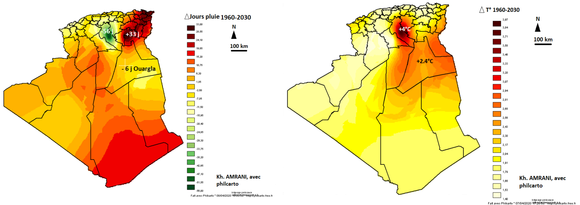
Figure 04 : Simulation du réchauffement climatique et de la variation du nombre de jour de pluie dans le Sahara algérien
