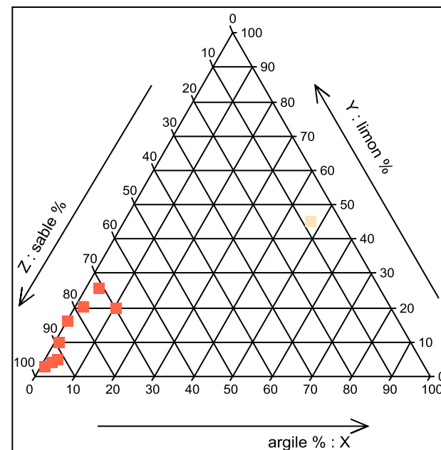
Figure 11 : Caractérisation des sols de Ouargla (Adapté d'après données auteurs et Omeiri, 2012)
