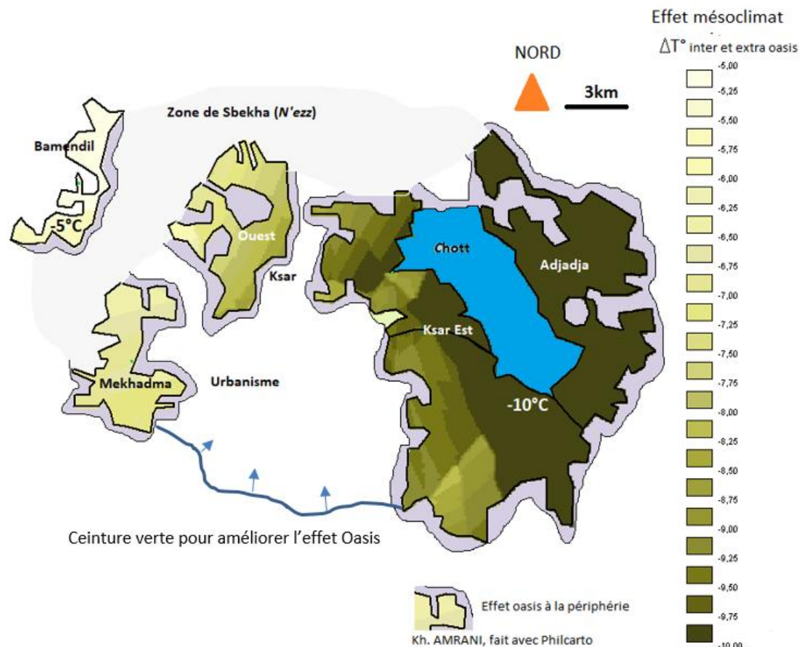
Figure 37 : Simulation de l'effet méso climatique dans la palmeraie de la cuvette de Ouargla (Données mesurées par Amrani, été 2018)
