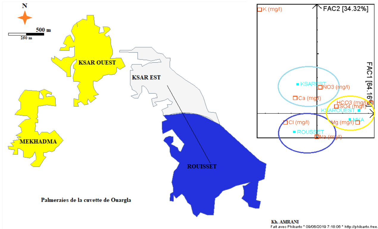
Figure 33 : Identification des sels responsables de la salinisation dans la cuvette de Ouargla (Auteurs selon les données de la figure 30)
