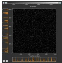
Ga planes (002) (004) (133)
