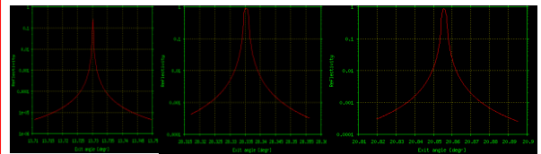
Ga planes (002) (004) (133)
