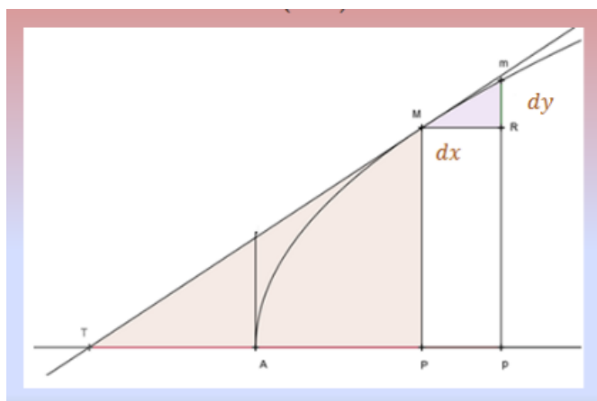
Figure 7 : Triangle caractéristique de côtés dx et dy semblable à TMP
