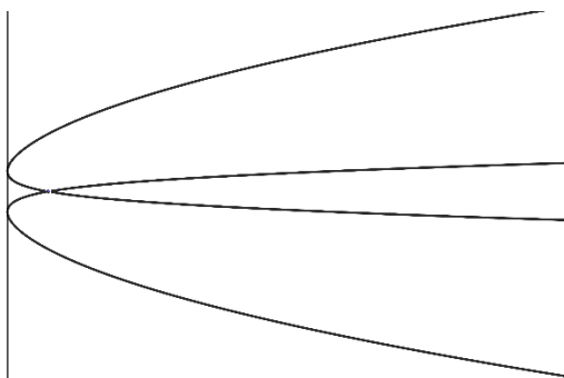
Figure 6 : Quartique d'équation y^4 - 8y^3 + 16y^2 - 12xy^2 + 48xy + 4x^2 - 64x = 0
