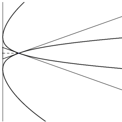
Figure 9 : Le deux sous-tangentes au point de décussation
