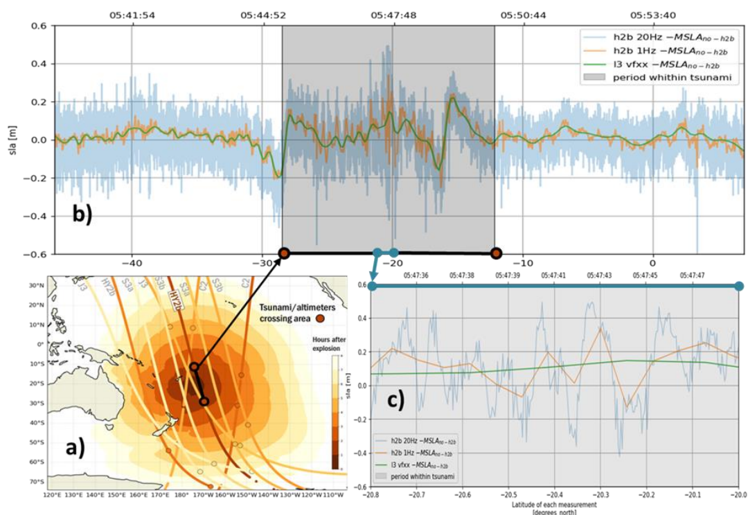
Figure 6 - Illustration de l'échantillonnage du tsunami par le satellite Haiyang 2B (HY2B). a) Colocalisation des prédictions de passage du tsunami (modèle fourni par le laboratoire Géozur) et de la constellation altimétrique. HY2B a été le premier satellite à survoler la zone, 1h30 après l'explosion, l'évènement ayant été mesuré ensuite par les autres satellites plus de 4 heures après l'explosion : Sentinel-3B (S3B), Cryosat-2 (C2), Jason-3 (J3), Sentinel-6A (S6A). b) Anomalie de niveau de la mer en utilisant les mesures à basse résolution (7 km) acquises par HY2B (en m) en fonction de la latitude sur l'échelle inférieure (unité en degré) et en fonction du temps sur l'échelle supérieure (unité en heure TU). La boîte grise correspond au segment noir du graphe a). A 28°S et 16°S, HY2B mesure de forts gradients proches des positions attendues dans le modèle. c) Zoom de l'anomalie de niveau de la mer
