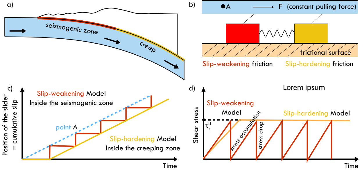
Figure 9. Modélisation d'une subduction en utilisant la méthode du patin-ressort. a) représentation schématique d'une subduction. b) Modèle conceptuel. c) Accumulation du glissement avec le temps. c) État de la contrainte cisailante au court du temps.
