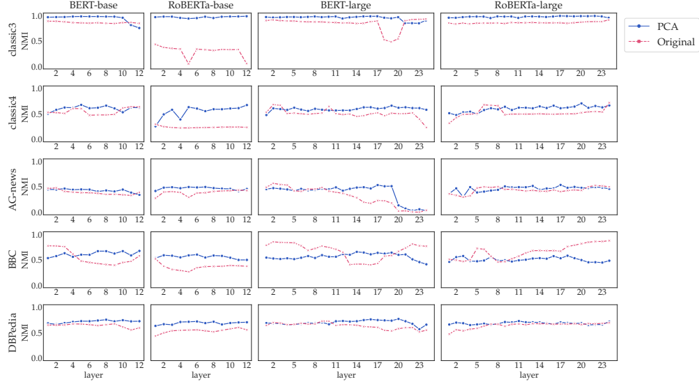
FIG. 3 – Performance du clustering (NMI) sur les représentations originales obtenues par chacune des couches des modèles pré-entraînés (en utilisant toutes les d dimensions des matrices \mathbf{X}^{(\ell)} ) par rapport aux représentations réduites ( d' = 100 ), avec \ell = 1, \dots, b .
