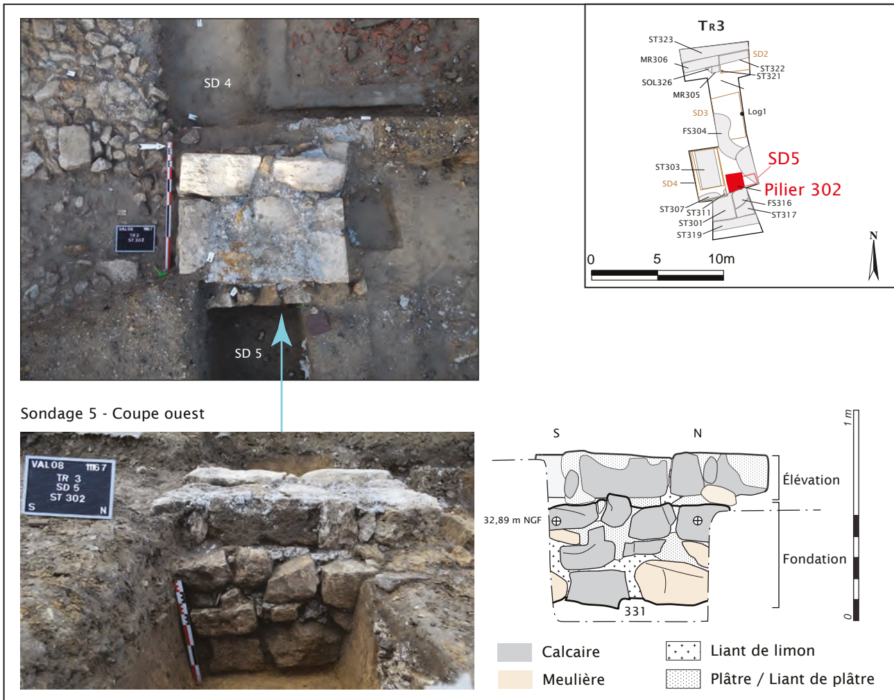
Figure 13 : Valenton, « La ferme de l'Hôpital quartier Val Pompadour » (Val-de-Marne). Coupes et photographies du pilier 302. © CD94, 2020.
