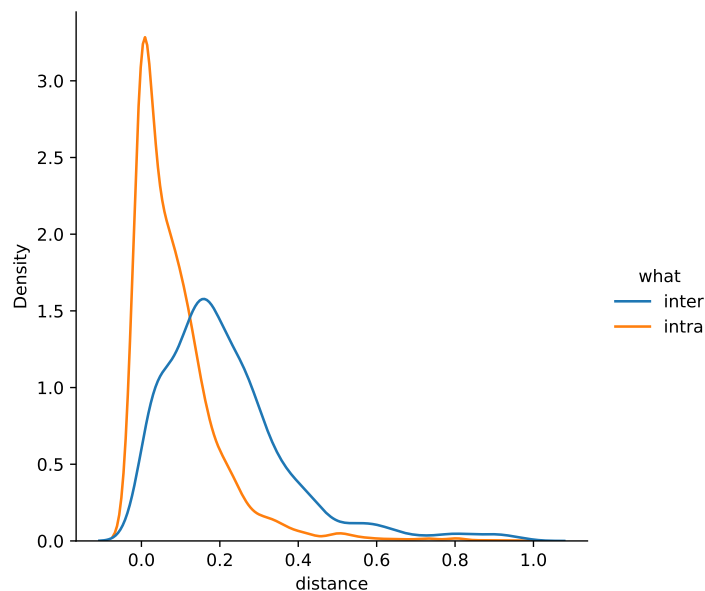
Figure 1: Distribution des distances d’éditation intra-système (entre les deux entraînements de JOEYNMT) et inter-système (entre les prédictions de JOEYNMT et de OPENNMT)
