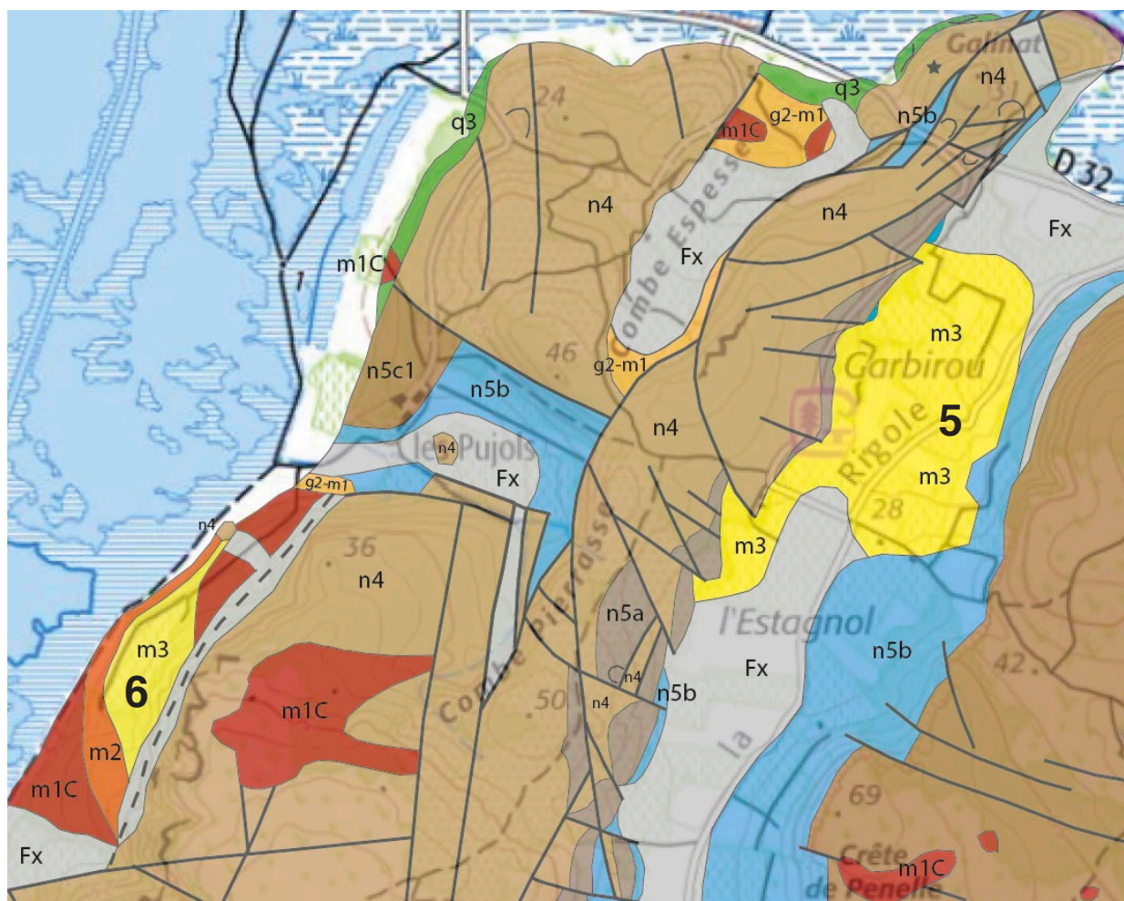
Fig. 8 – Les affleurements de Miocène (m3) du centre et de la façade occidentale de l'Île Saint-Martin. Aggrandissement de la carte géologique (leviers personnels). 5. Garbirou ; 6 : Sud des Pujols. Même légende que celle de la Fig. 3.
