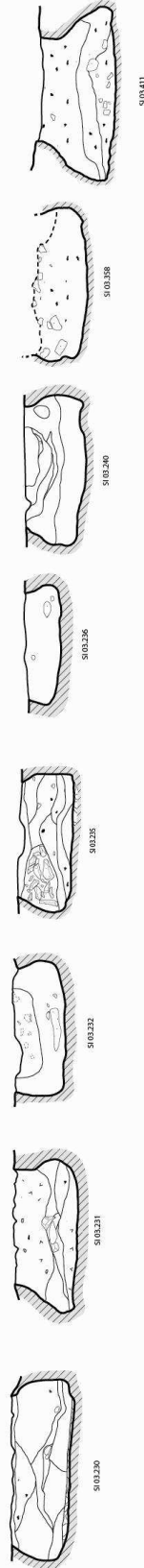
Type 2 : Silos tronconiques
