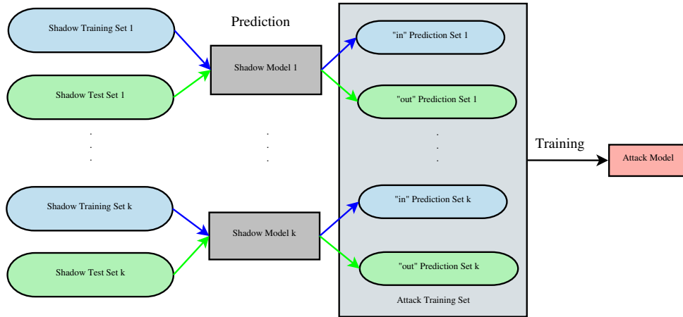
FIG. 6 – Création du modèle d'attaque par inférence.
