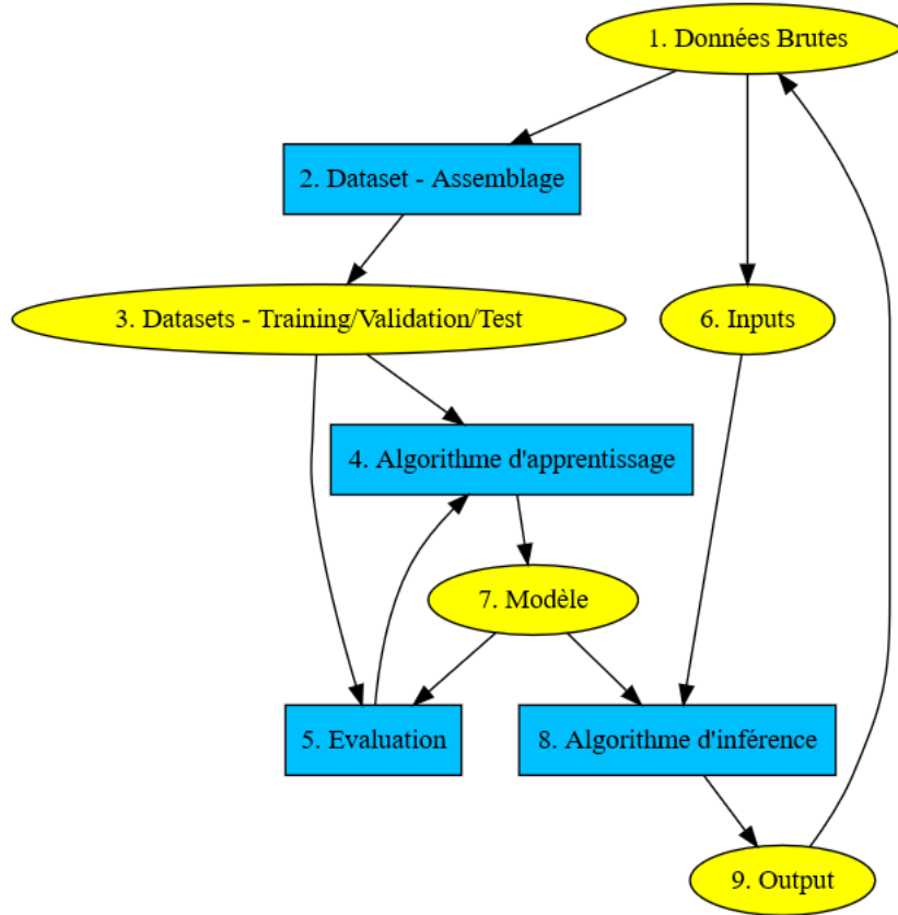
FIG. 1 – Framework de l'apprentissage automatique.
