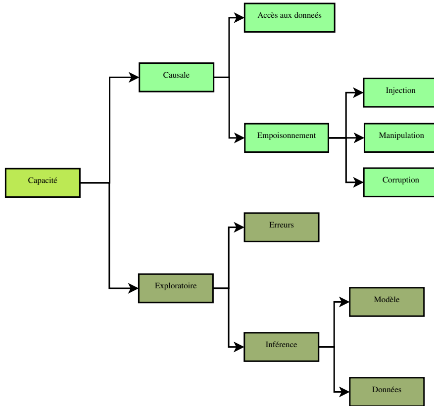
FIG. 5 – Capacité de l'attaquant.
