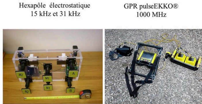
Fig. 11. Dispositifs d'investigation décamétrique utilisés pour les murs : Hexapôle électrostatique où la voie 1 prend en compte une épaisseur de 8 à 10 cm et la voie 2 une épaisseur de 15 à 20 cm et Radar 'Pulse Ekko' (Sensors and Software) de fréquence centrale 1 GHz.
