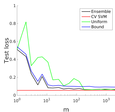
(d) Waveform dataset. n = 2000 , r = d + 1 = 41 .
