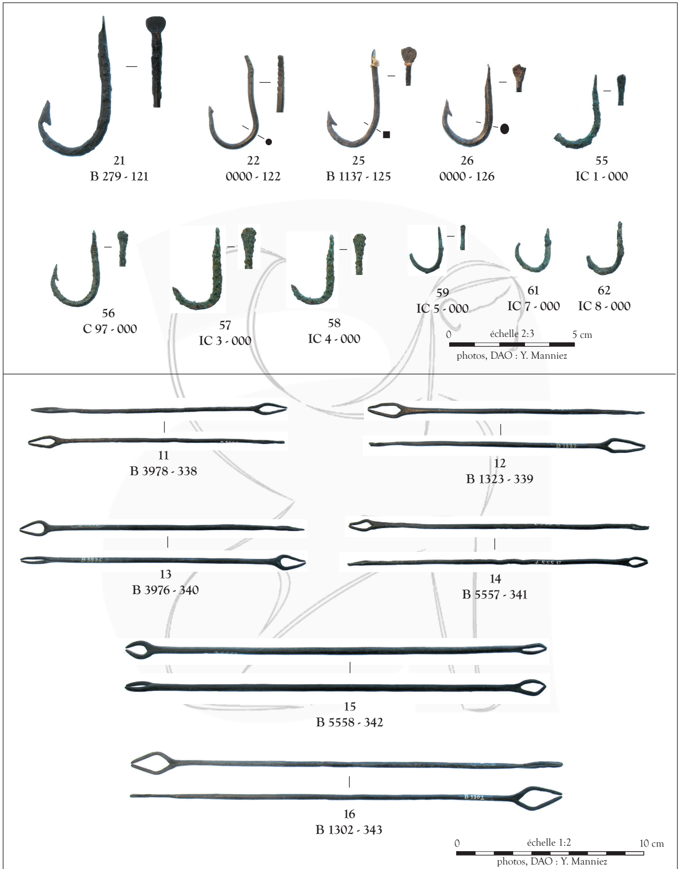
Fig. 3. Les hameçons (suite) et les navettes à filet (DAO. Y. M.).
