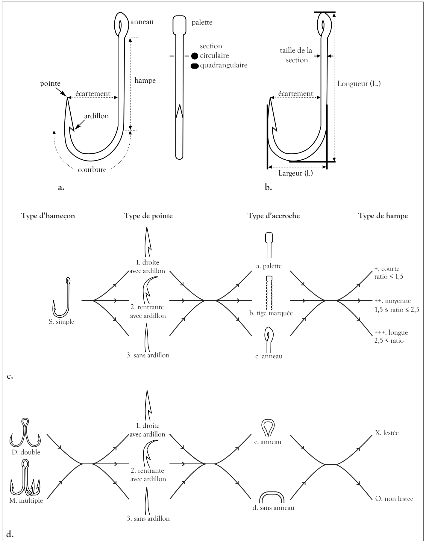
Fig. 30. Terminologie des hameçons (a.), prises de mesures (b.) et proposition de typologies pour les hameçons simples (c.), doubles et multiples (d.) (DAO B. E.).
