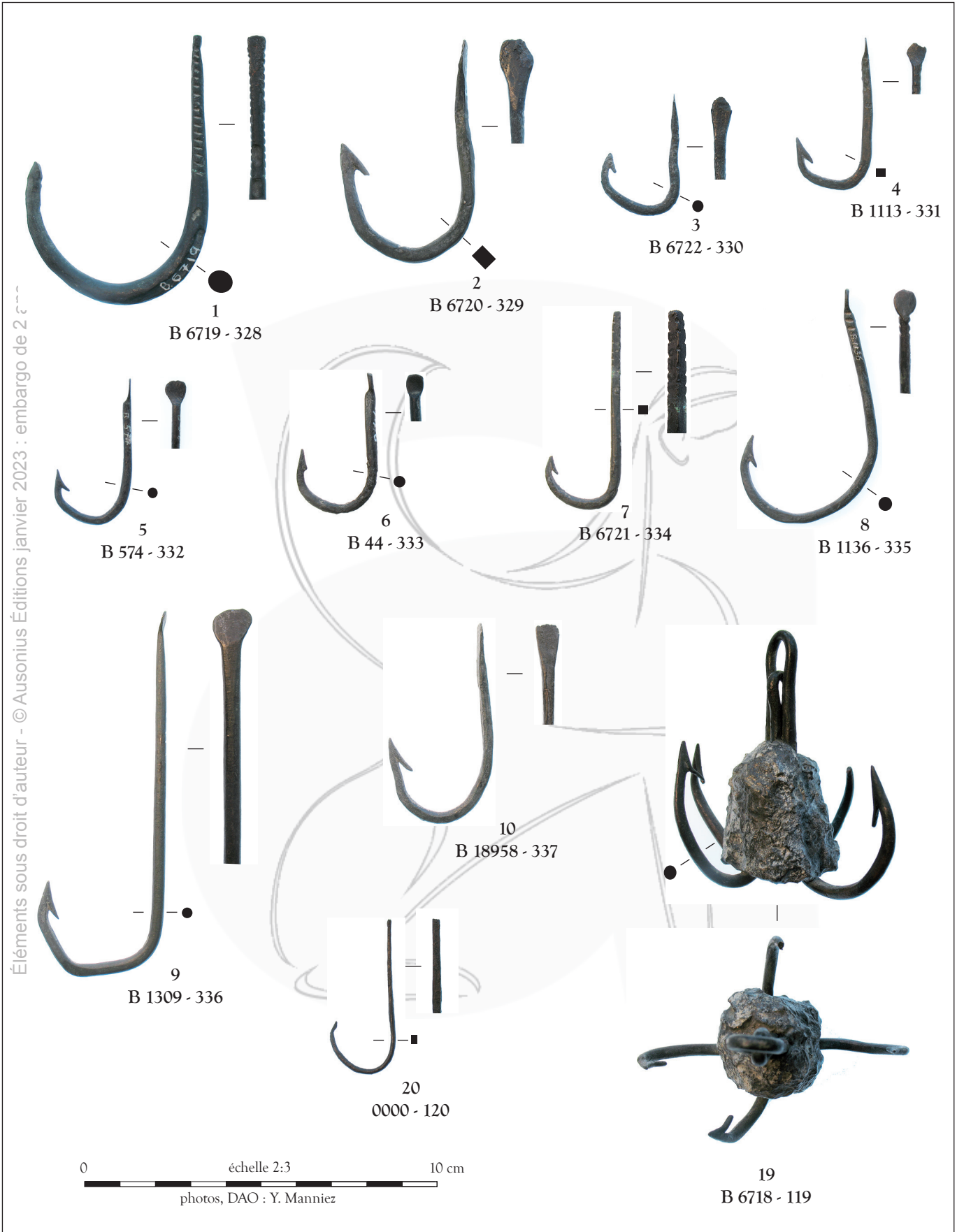
Fig. 2. Les hameçons (DAO. Y. M.).
