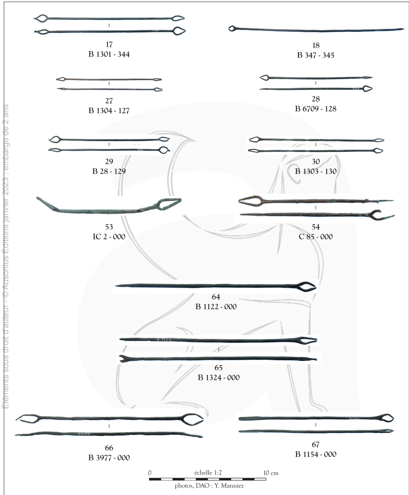
Fig. 4. Les navettes à filet (suite) (DAO, Y. M.).
