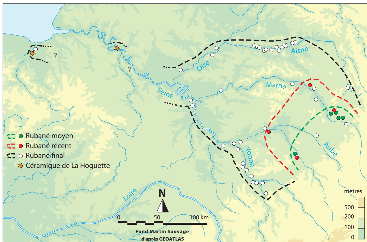
Fig. 1 – Répartition des sites d’habitat datés du Rubané dans le Bassin parisien. Les découvertes isolées de céramique de La Hoguette sont indiquées également. Les traits en pointillé montrent l’extension de la colonisation par grandes étapes chronologiques. Les appellations Rubané moyen, récent et final correspondent à la nouvelle terminologie proposée ici.
