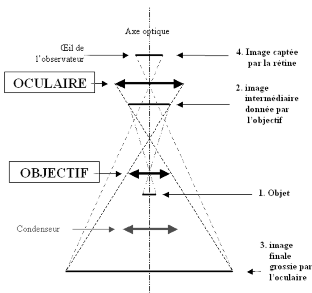
Figure 81 : Principe de la microscopie optique.
