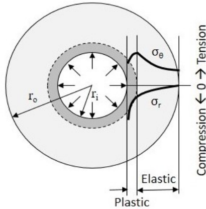
(d) After autofrettage [47]
