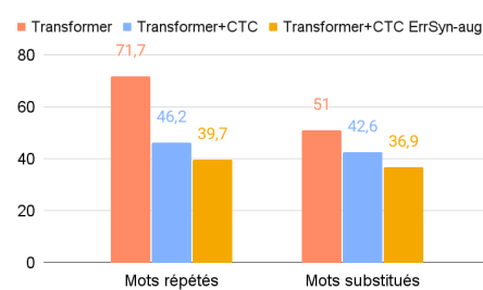
FIGURE 2 – PER (%) du Transformer, Transformer+CTC et Transformer+CTC ErrSyn-aug pour les mots répétés ou substitués
