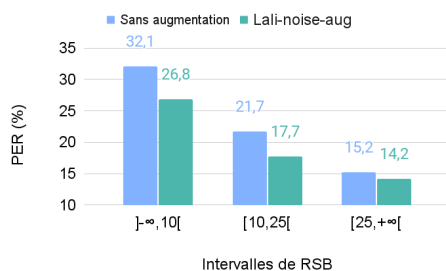
FIGURE 1 – PER (%) du Transformer+CTC avec et sans augmentation Lali-noise , pour différents intervalles de RSB
