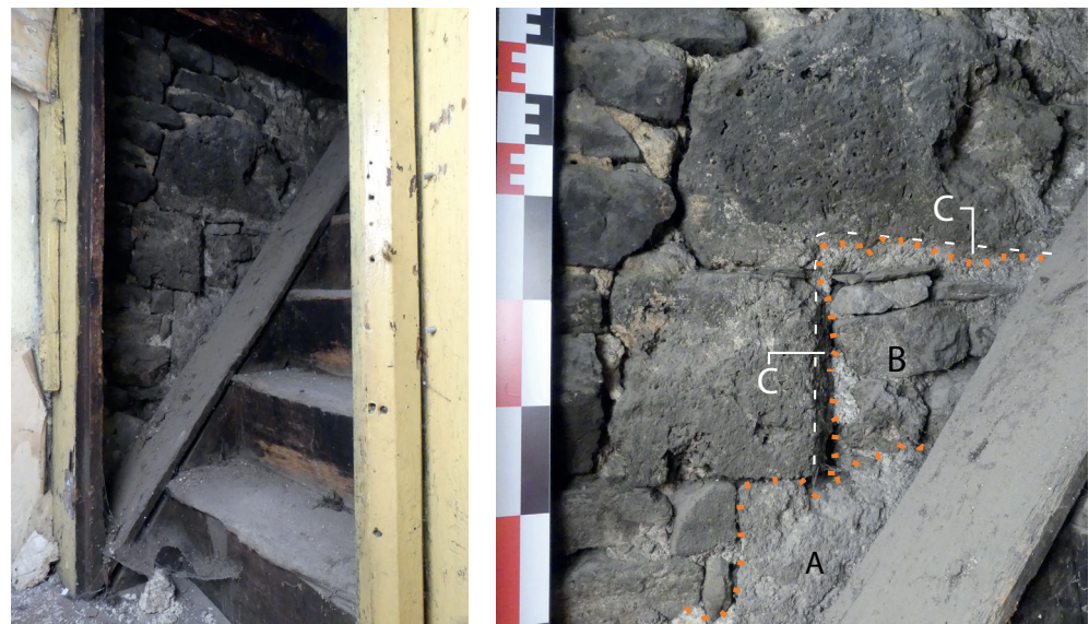
fig. 18 Les maçonneries dans l'angle sud-ouest de la maison du 5 place du Mazel, au 1 er étage, sous la cage d'escalier montant au 3 e . La vue est prise du nord-est. À droite, le mur MR1007 de la maison voisine de l'ouest et à gauche la façade méridionale MR1001 (ici US 1023) évidée d'une niche. A : chaînage d'extrémité du mur MR1001. B : maçonnerie d'obturation de fenêtré.
