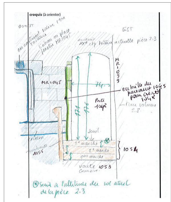
1048 - Croquis de l'élévation de la porte 1048 du mur MR1045, face externe (côté loggia L01056)
