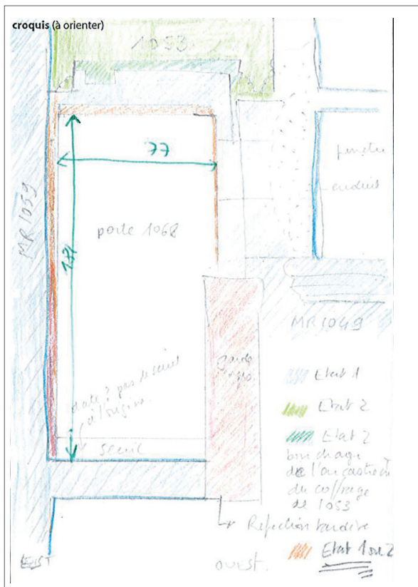
1068 - Croquis de l'élévation de la porte 1068 du mur MR1049, face externe (côté loggia LO1077)
