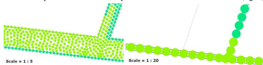
Figure 6. Représentation de la quantité de chlore soit dans la canalisation, soit sur l'axe de la canalisation selon le niveau de détail.
