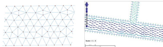
Figure 1. Extrait du TIN pour l'écoulement et Représentation des vitesses
