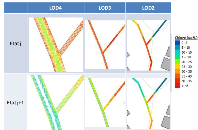
Figure 14 Diffusion de chlore dans la canalisation : 2 états consécutifs à 3 LoD.
