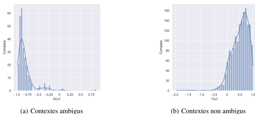
Figure 3. Distributions de r et b sur les phrases de notre corpus
