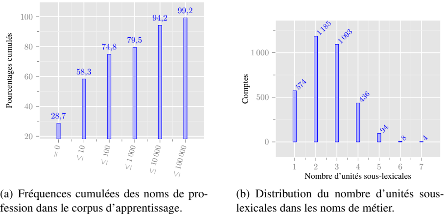
Figure 1. Rareté des noms de profession dans le corpus d'apprentissage
