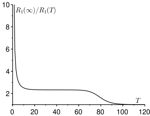
Figura 4.3: Il rapporto R_1(\infty)/R_1(T) in funzione di T .
