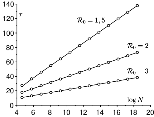
Figura 1.4: Il momento \tau di occorrenza del picco epidemico del modello S-I-R, in giorni dall'inizio dell'epidemia, in funzione di \log N secondo la formula esatta (1.9) [linee solide] e secondo la formula approssimata (1.10) [piccoli cerchi]. Valori dei parametri: I_0 = 1 , b = 1/4 al giorno, \mathcal{R}_0 = a/b \in \{1,5; 2; 3\} .
