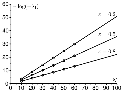
Figura 19.2: Calcolo dei moltiplicatori di Floquet dell'equazione principale: -\log(-\lambda_1) in funzione di N per \varepsilon = 0,2, 0,5 o 0,8 e N = 10, 20, \dots, 60 . I valori di C sono rappresentati dalle pendenze di queste linee. Valori dei parametri: T = 1, a_0 = 20, b = 5 .
