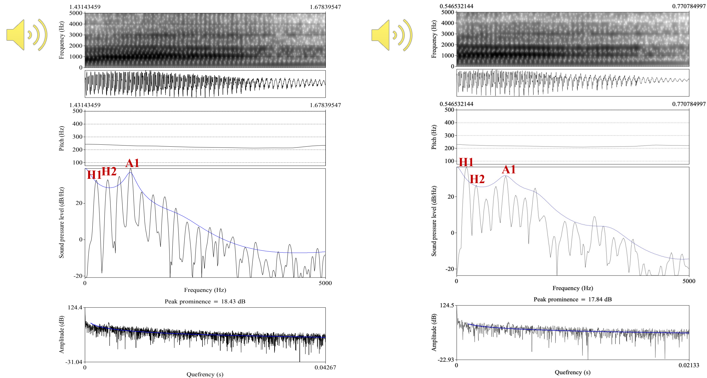
FIGURE 8 : Spectrogramme, signal, contour F0, spectre (1 er intervalle de la durée vocalique), cepstre du mot « pas » produit avec une voix moins soufflée (à gauche) et une voix plus soufflée (à droite) par une locutrice du wu
