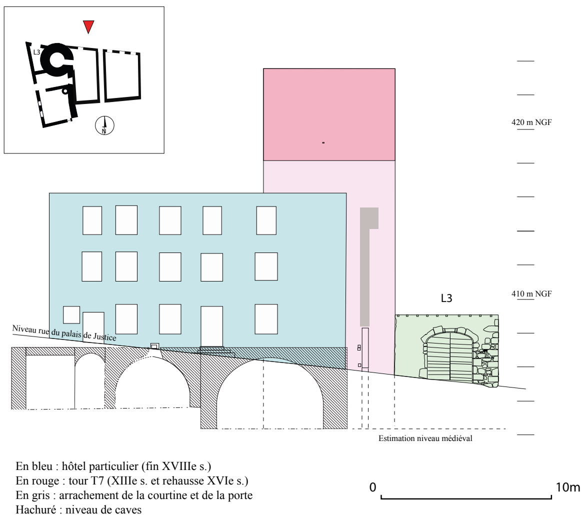
Figure 14 : Elevations sur la rue du Palais de Justice.
