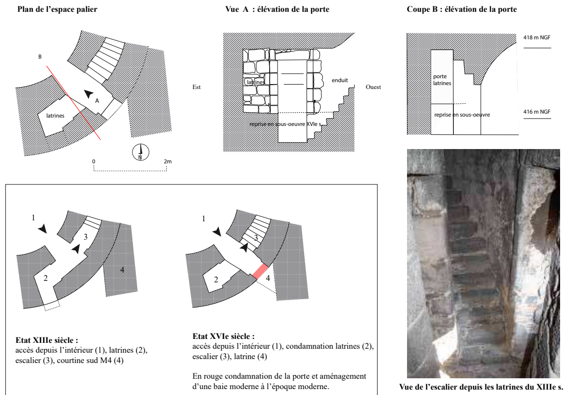
Figure 12 : Relevés et plan de l'espace palier de la tour
