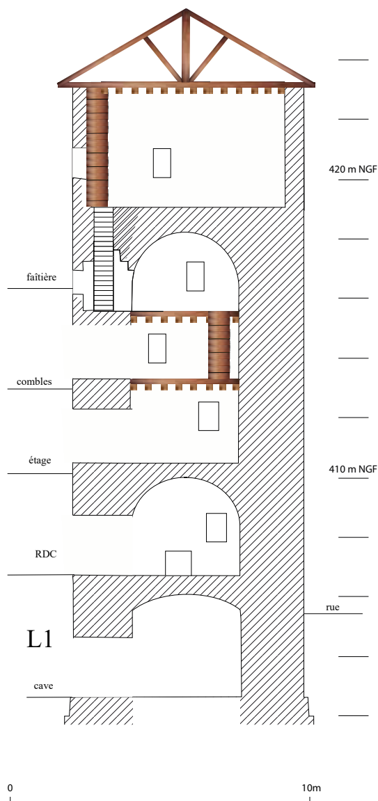
Figure 5 : Coupe de la tour (Relevés C.M).
