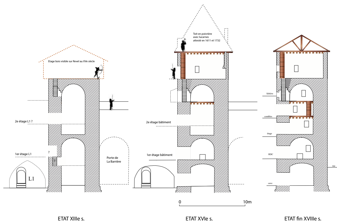
Figure 24 : Evolution de la tour de La Barrière entre le XIIIe et le XVIIIe siècle.
