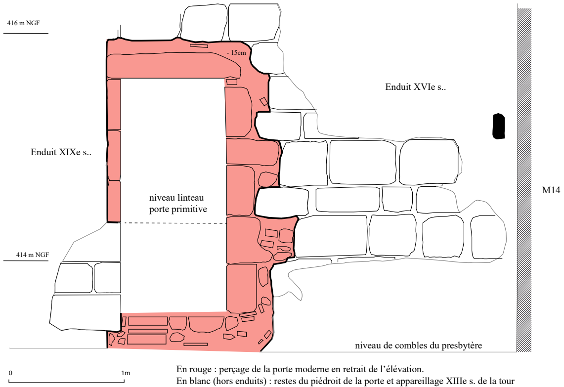
Figure 11 : Relevé d'élévation de la porte d'accès à la partie supérieure de la tour depuis L1.
