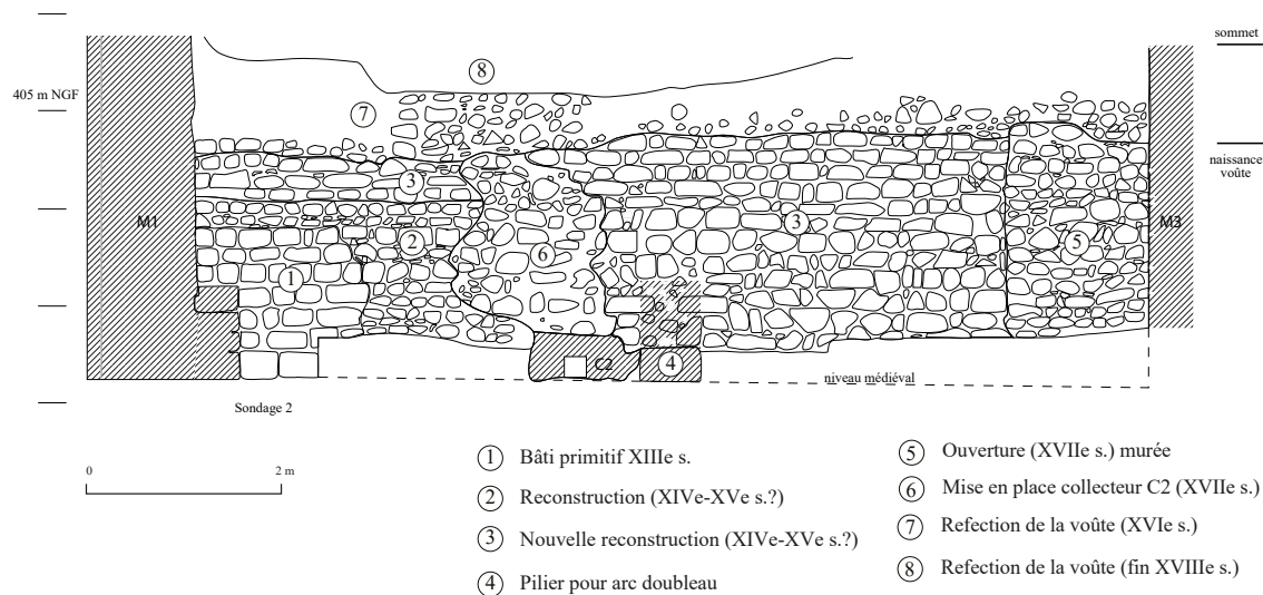
Figure 20 : Elévation orientale (M4) de L1.
