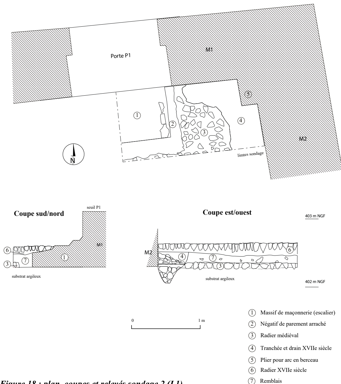
Figure 18 : plan, coupes et relevés sondage 2 (L1).
