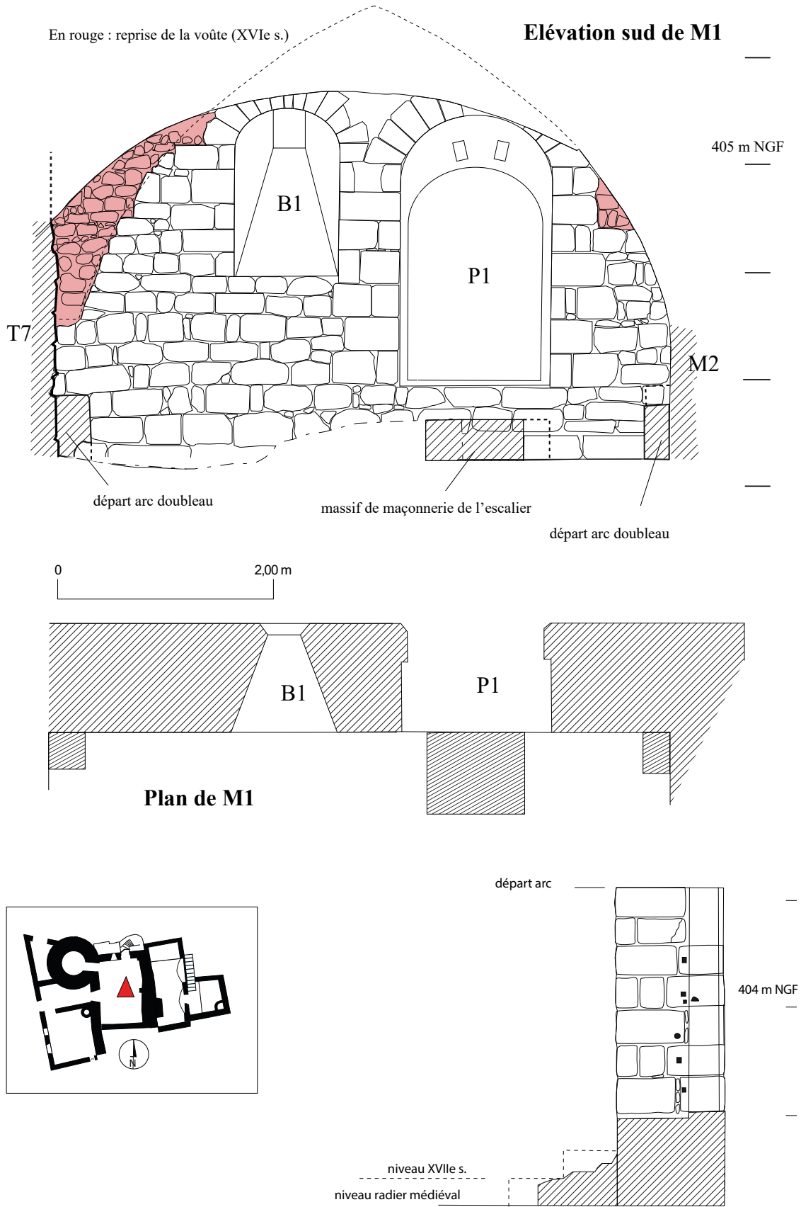
Figure 17 : plan, coupe et relevés du mur M 1 (L 1).
