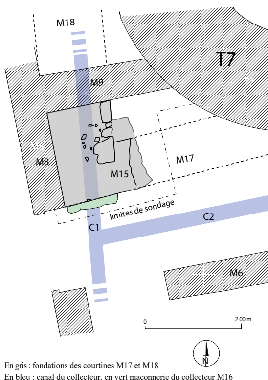
Figure 15 : Plan des structures du sondage 1.
