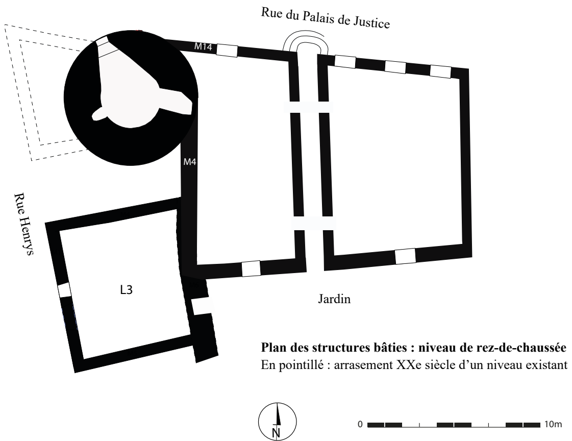
Figure 4 : Plan de l'ensemble immobilier du 14 rue du Palais de Justice.
