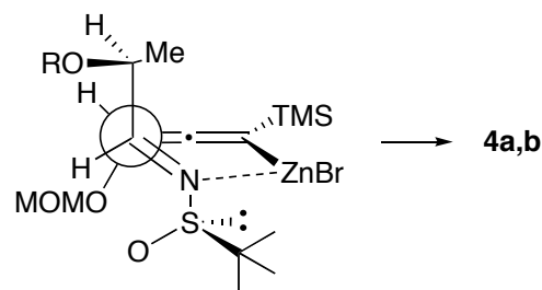
TS1 (Felkin) : R = TBS, Bn
